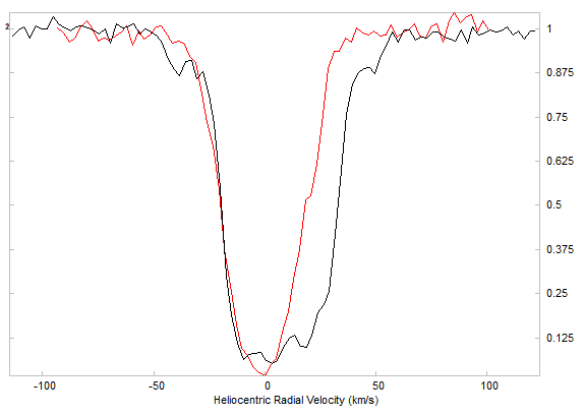
Рисунок 2.8. Профили линии K (3933.633 Å) межзвездного Ca II звезд BD -13 4927 (красный) и BD -13 4929 (черный). На небе их разделяет ~3 угловые минуты.
