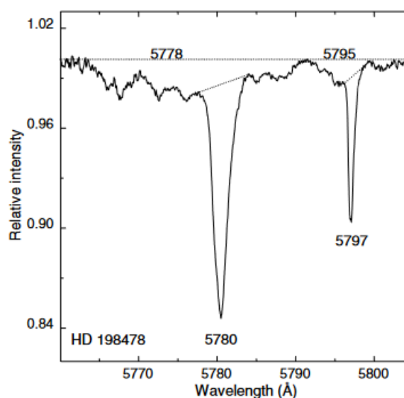
Рисунок 1.6. ДМП 5780 и 5797 в спектре звезды HD 198478 блендированы широкими ДМП 5778 и 5795 соответственно. Прерывистая линия указывает на уровень псевдо-континуума для корректного измерения эквивалентных ширин полос 5780 и 5797.
