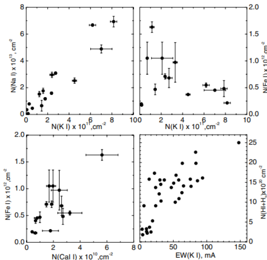
Рисунок 2.39. Корреляции между лучевыми концентрациями разных компонент МЗС в объектах исследования.
