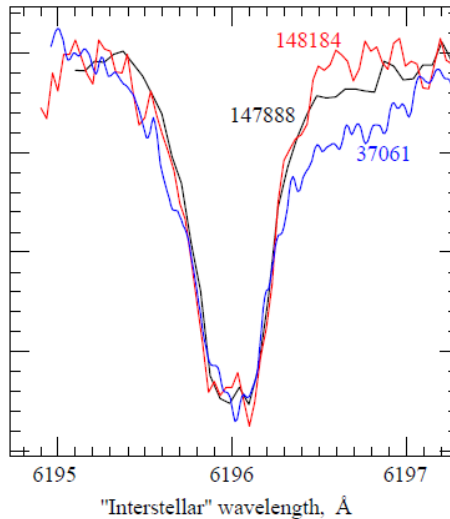
Рисунок 1.14. Переменность профиля ДМП6196.
