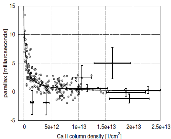
Рисунок 2.6. Соотношение параллакс – лучевая концентрация. Для наглядности показаны только самые большие значения ошибок. Аппроксимирующая функция показано жирной сплошной линией.
