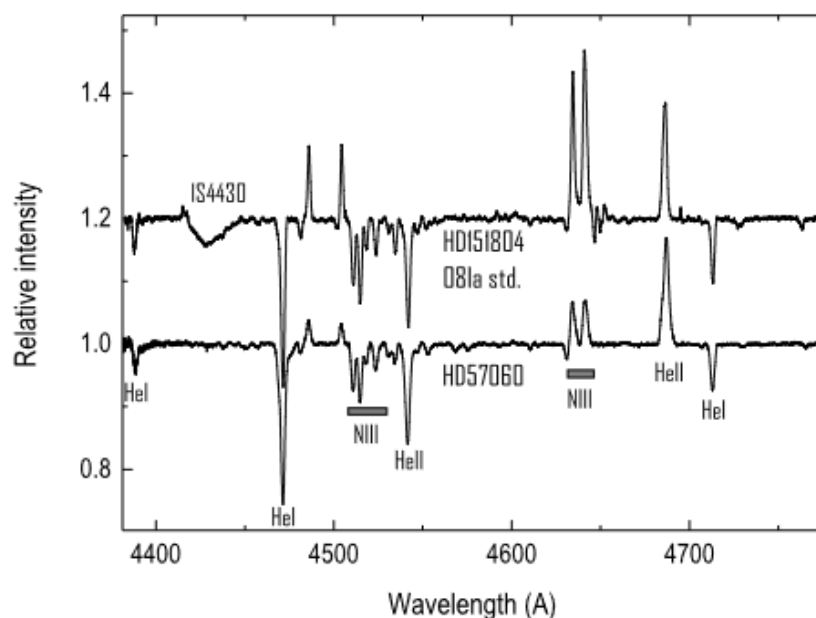
Рисунок 4.10. Спектр HD 57060 в сравнении с HD 151804 – стандартом O8Ia, согласно Walborn & Fitzpatrick, (1990).
