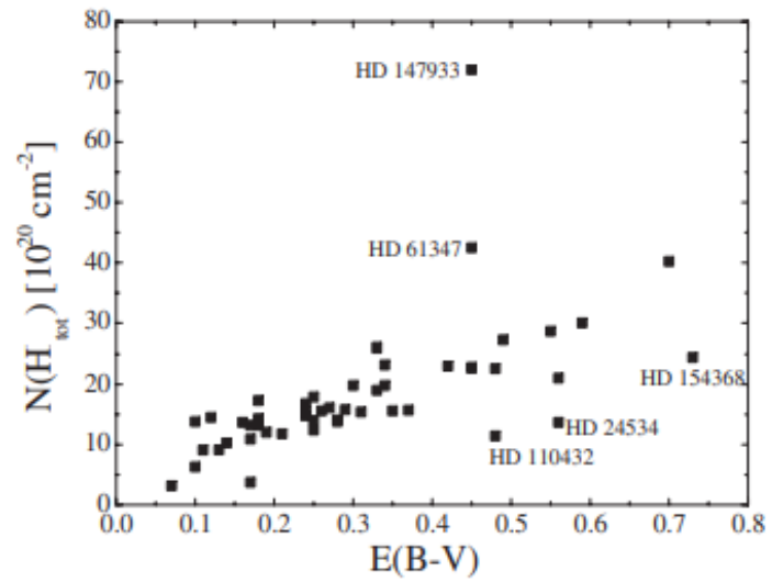
Рисунок 3.17. В отличие от N(\text{CH}^+) , водород, как атомарный, так и молекулярный демонстрирует относительно высокую корреляцию с межзвездным покраснением.
