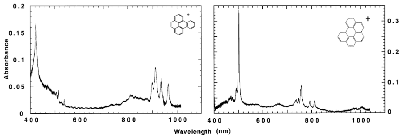
Рисунок 5.56. Абсорбционные спектры катионов ПАУ C_{20}H_{12}^+ (слева) и C_{22}H_{12}^+ (справа), полученные в неоновой матрице.
