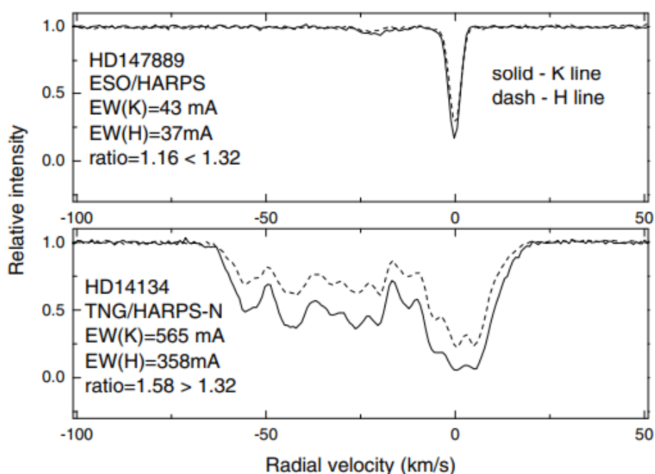
Рисунок 2.20. Пример того, что облака, видимые в компонентах профилей дублета Ca II и, наблюдаемые в направлении l = 135^\circ , равномерно заполняют диск Галактики: количество компонентов растет с расстоянием, каждый последующий все больше смещается в голубую сторону (нижний рисунок). Благодаря этому многие компоненты профилей H и K остаются свободными от сильного насыщения, в то время как насыщение может быть очевидным даже для близлежащих объектов (верхний рисунок.)
