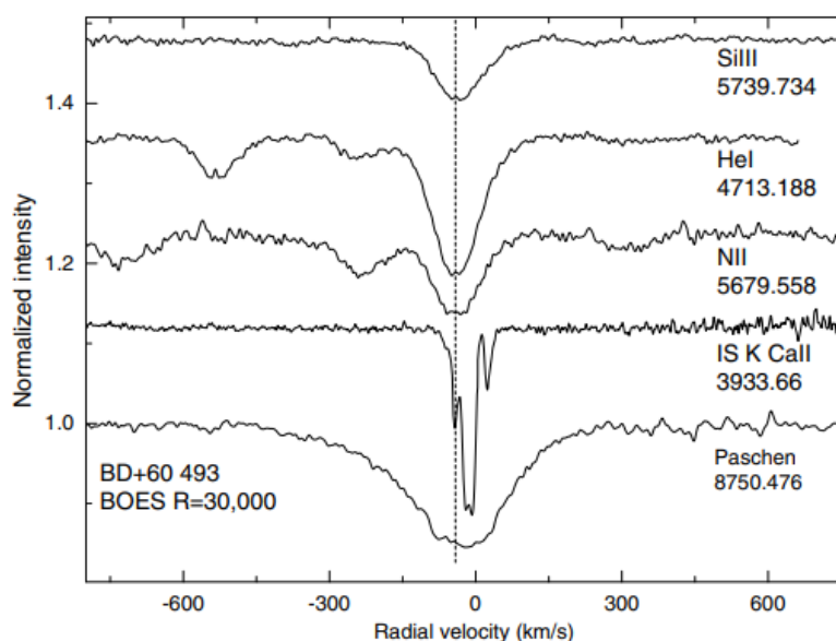
Рисунок 2.21. Профили линий звезды в направлении l = 135^\circ и профиль межзвездной линии Ca II в спектре BD +60 493. Компоненты межзвездных профилей образованы облаками, расположенными между наблюдателем и звездой, т. е. звезда является самым удаленным объектом. Лучевая скорость самого дальнего облака (ближайшего к звезде), отмеченная вертикальной пунктирной линией, примерно совпадает со скоростями фотосферных линий.
