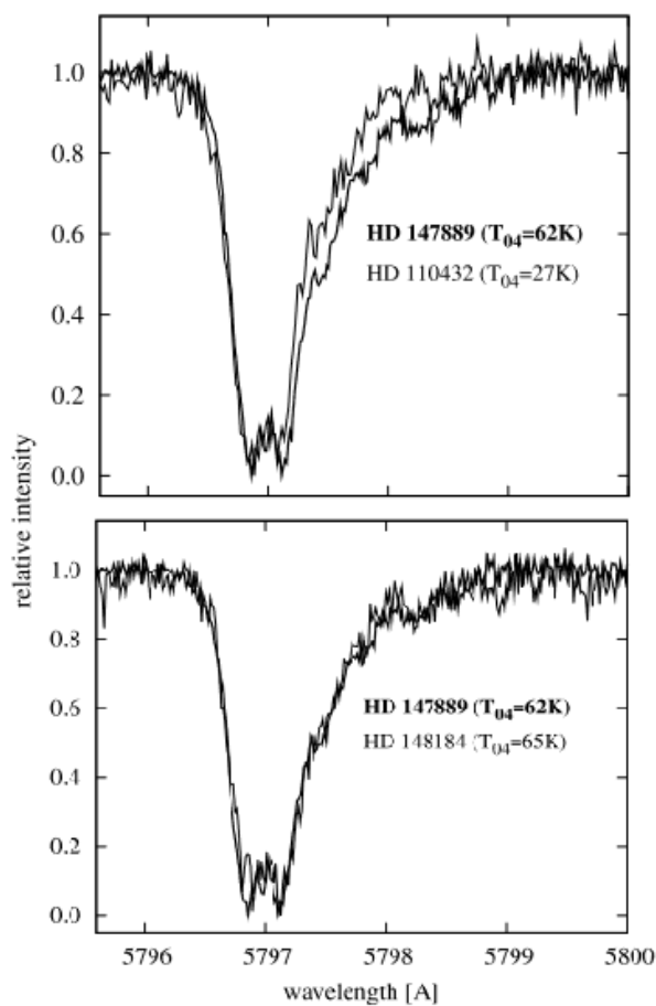
Рисунок 5.30. Нормализованные по интенсивности (для наглядности) профили ДМП 5797 Å. Ширина профиля зависит от температуры возбуждения T_{04} молекулы C_2 .
