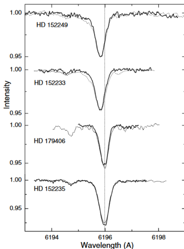
Рисунок 1.8. «Голубой» сдвиг ДМП 6196 в двух объектах ассоциации Sco OB1, подтвержденный спектрами с двух инструментов: жирная линия – HARPS, тонкая прерывистая – Feros.
