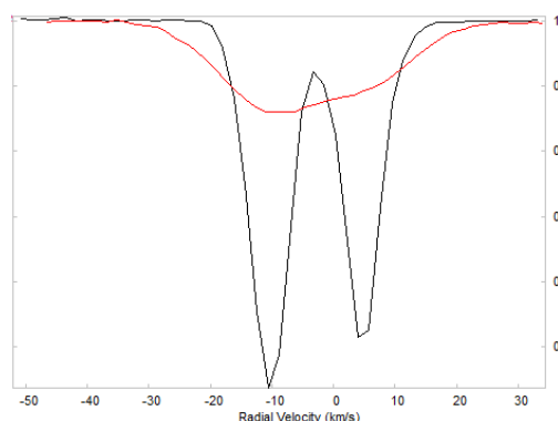
Рисунок 5.74. Профили межзвёздного калия 7699 Å и ДМП 6196 HD 183143 в шкале лучевых скоростей.
