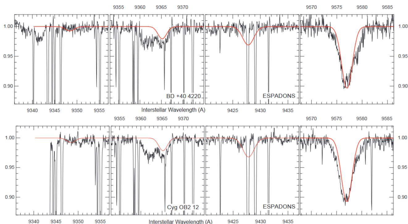
Рисунок 5.84. Диффузные полосы показаны вместе с гауссианами, которые имитируют положения, ширину и относительную интенсивность лабораторных линий по данным Campbell et al. (2016). Обратите внимание на отсутствие межзвездных абсорбций на месте линии C_{60}^+ 9428 Å.
