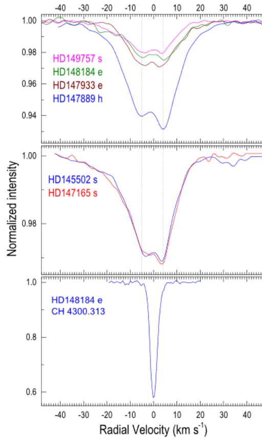
Рисунок 5.50. Расщепленные профили ДМП 6196 Å. Вертикальные пунктирные линии (между ними 9 км/с) показаны для наглядности.
