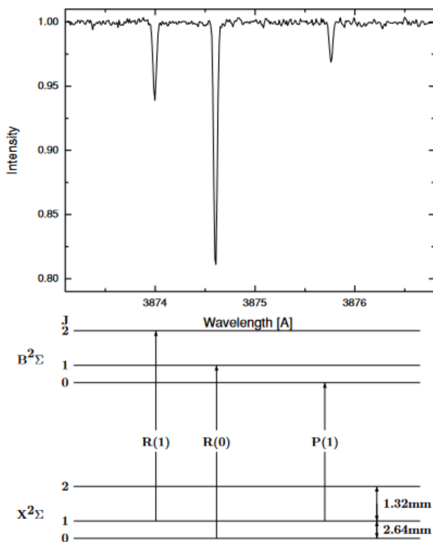
Рисунок 3.21. Диаграмма термов полосы B^2\Sigma^+ - X^2\Sigma^+ (0,0) молекулы CN с соответствующим фрагментом спектра в направлении на HD147889, полученном с помощью спектрографа HARPS (R=115000).
