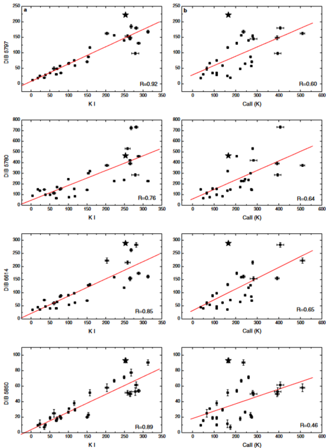
Рисунок 5.25. Исследование связи эквивалентных ширин ДМП 5850, 6614, 5780 и 5797 с калием и ионизованным кальцием. Коэффициент корреляции указан на каждом графике справа внизу. Звездочкой обозначен пекулярный случай HD186745 (экстремальный \zeta объект).
