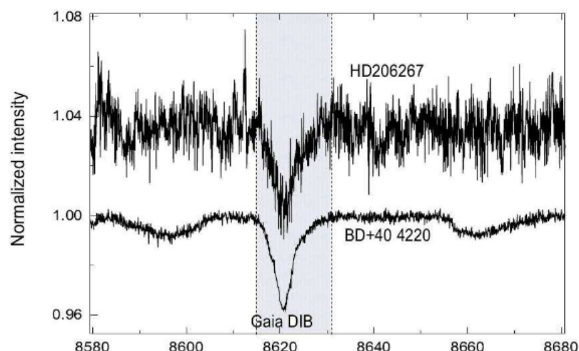
Рисунок 5.21. Иллюстрация метода, который мы применили для измерения эквивалентной ширины ДМП 8620 в спектрах с низким S/N. Профиль ДМП 8620 с высоким отношением S/N (в спектре BD+40 4220) служит шаблоном и нормируется для соответствия глубине этой же ДМП в спектре HD 206267. Затем измеряется эквивалентная ширина шаблона. На рисунке спектры разнесены по вертикали для наглядности. Для справки: EW_{8620}(BD+40\ 4220) = 701 \pm 24\ \text{mÅ} , EW_{8620}(HD\ 206267) = 205 \pm 48\ \text{mÅ}
