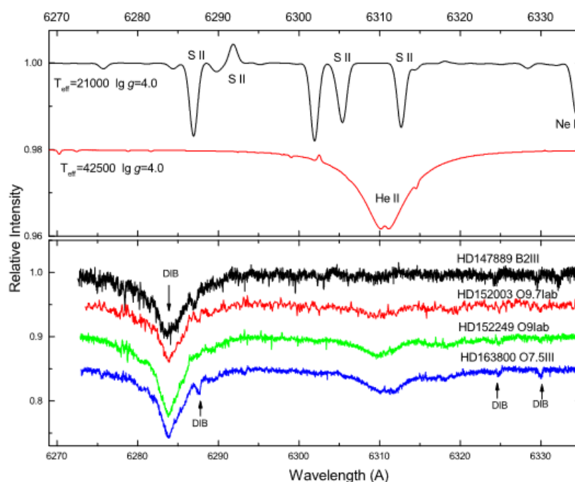
Рисунок 5.8. Спектральная особенность, упомянутая как возможная ДМП 6311 в работе Sonnentrucker et al. (2018), на самом деле является звездной линией He II, характерной для звезд O-типа.
