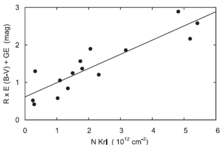
Рисунок 4.5. Соотношение между лучевой концентрацией межзвездного криптона и полным поглощением, включающем R \times E(B-V) и GE. Средняя ошибка лучевой концентрации криптона составляет около 15 процентов.
