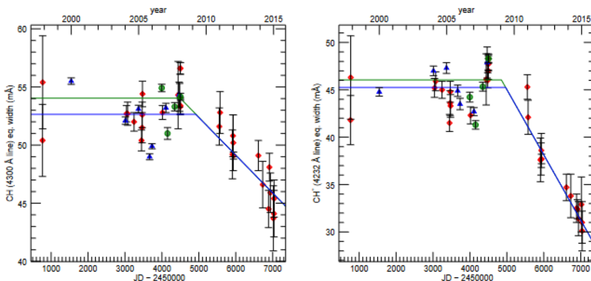
Рисунок 5.42. Изменение эквивалентной ширины линий CH 4300 Å (слева), CH+ 4232 Å (справа) с временем (внизу юлианские даты, сверху - годы). Эквивалентная ширина у линии CH+ падает быстрее чем у CH. Красные точки — наши измерения, синие и зеленые точки из Boissé et al. (2009).
