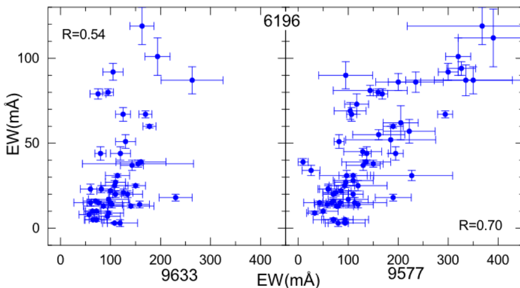
Рисунок 5.85. Сравнение эквивалентных ширин ДМП 9577, 9633 и узкой диффузной полосы 6196. Указан коэффициент корреляции.
