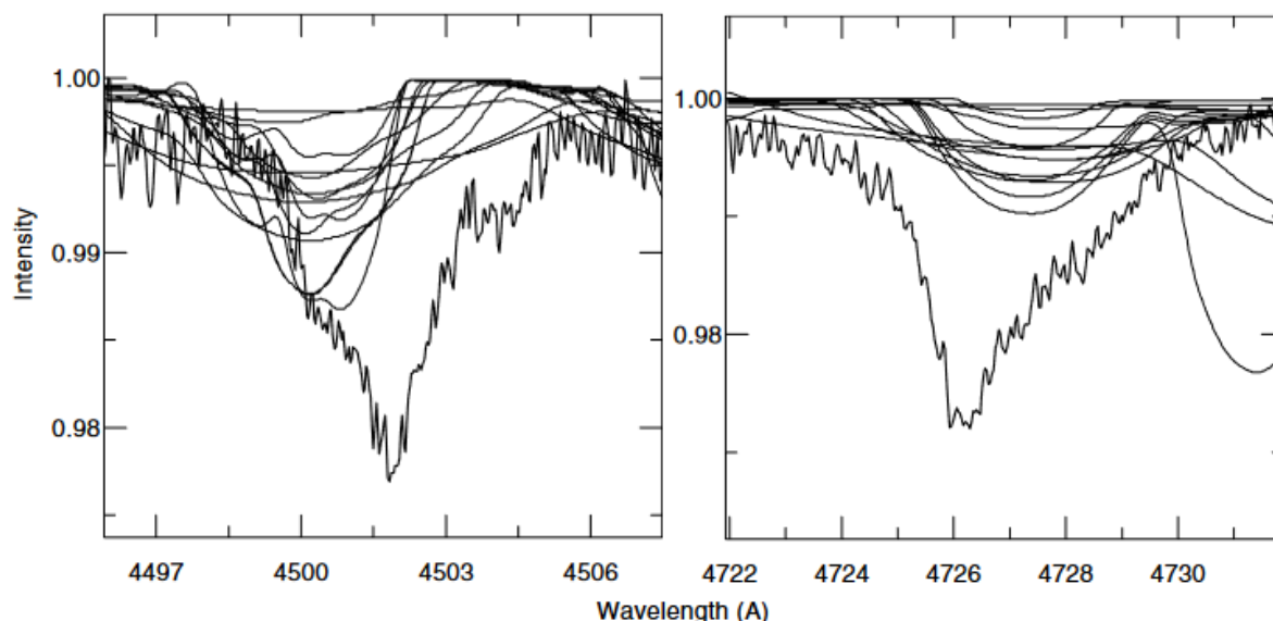
Рисунок 5.16. (Слева) Профиль ДМП 4502 полученный усреднением спектров 26 звезд с набором кривых соответствующих синтетических спектров. Сложный профиль ДМП может быть результатом вклада звездных линий. (Справа) То же самое для ДМП 4726. Очевидная асимметрия профиля, как минимум, частично обусловлена влиянием звёздных линий.
