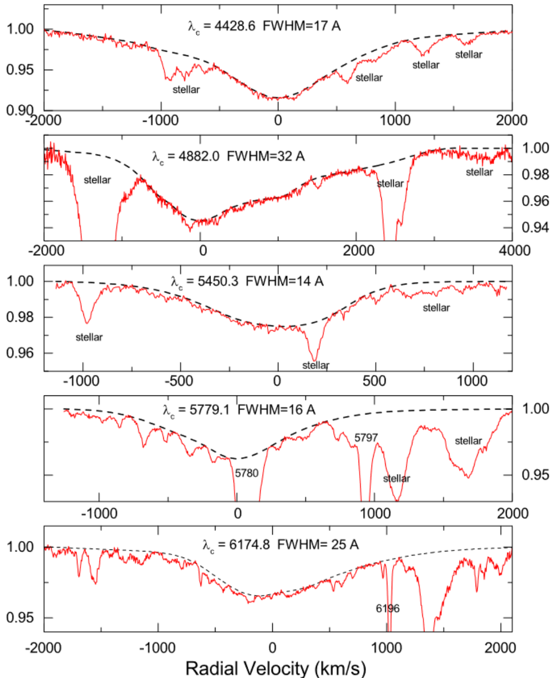
Рисунок 5.13. Усредненные для всех объектов профили широких ДМП в межзвездной шкале лучевых скоростей. Даны длина волны покоя и FWHM. Все неотмеченные абсорбции являются диффузными полосами (см. рисунок 5.9).
