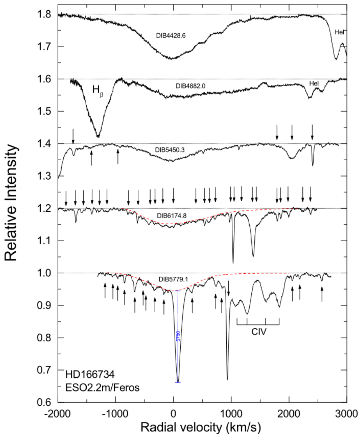
Рисунок 5.9. Профили подтвержденных широких ДМП в спектре горячей двойной О-звезды. Стрелки отмечают узкие диффузные полосы. Пунктирные красные линии показывают профили широких ДМП 6175 и 5779. Обратите внимание на вертикальную линию внутри профиля ДМП 5780, обозначающую интенсивность (глубину) этой ДМП.
