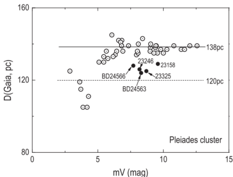
Рисунок 2.32. Параллаксы членов Плеяд относительно видимого блеска. Две параллельные горизонтальные линии показывают: (вверху) — параллакс GAIA DR2 всех показанных звезд и (внизу) — средний параллакс, полученный на основе измерений Hipparcos (van Leeuwen, 2009). Обратите внимание на совпадение результата Hipparcos с положением самых ярких звезд на рисунке.
