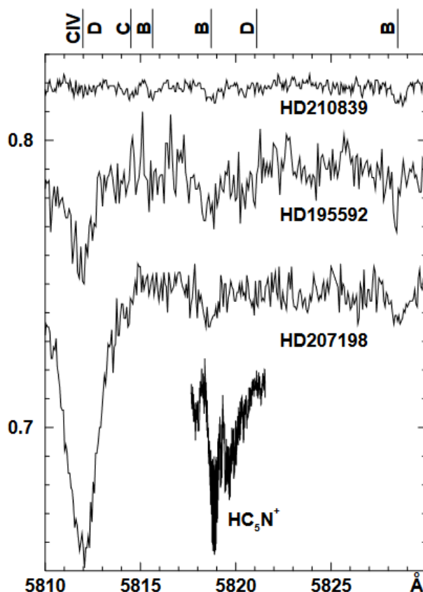
Рисунок 5.51. Лабораторный спектр молекулы \text{HC}_5\text{N}^+ в газовой фазе и спектры трех покрасневших звезд.
