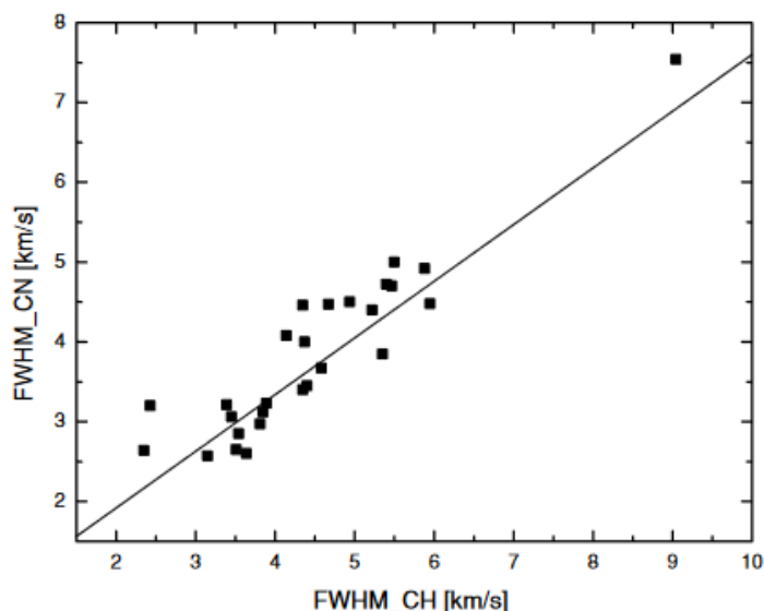
Рисунок 3.25. Сравнение ширины профилей линий молекул CN и CH. Наклон аппроксимирующей кривой соответствует отношению массы частиц и указывает на то, что турбулентная скорость газа не играет существенной роли: параметр b молекулы CH можно перемасштабировать для молекулы CN как b_{\text{CN}} = b_{\text{CH}}/\sqrt{2} .
