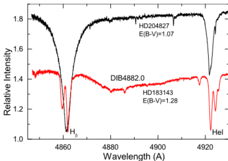
Рисунок 5.7. Фрагменты двух спектров сильно покрасневших звезд. Обратите внимание на отсутствие прямой связи между интенсивностью ДМП 4882 и покраснением E(B-V) .
