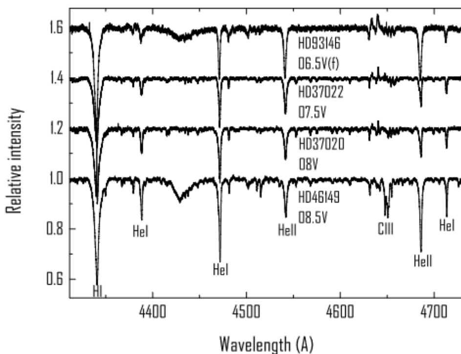
Рисунок 4.7. Спектры HD 37022 и HD 37020 со стандартами Walborn & Fitzpatrick (1990). Спектральный класс O-звезд определяется по отношению интенсивности линий He I/He II. Широкие профили линий водорода у звезд Ориона подтверждают, что они являются карликами.
