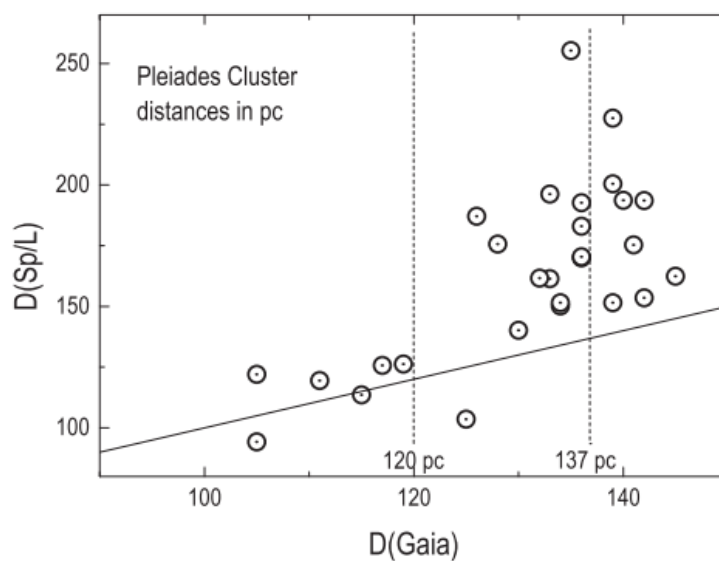
Рисунок 2.35. Сравнение расстояний до ярких членов Плеяд полученных двумя методами. Обратите внимание на значительное отклонение спектрофотометрических расстояний от линии совпадения (прямая на графике) для звезд, близких к основной части скопления (137 пк). Также указано среднее расстояние до скопления по Hipparcos (120 пк).
