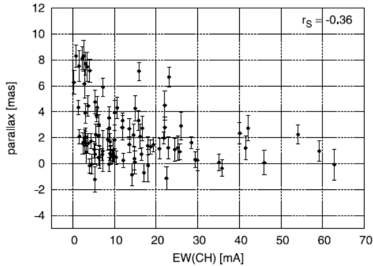
Рисунок 2.3. То же самое, что и на рисунке 2.1, но для линии CH 4300.321 Å
