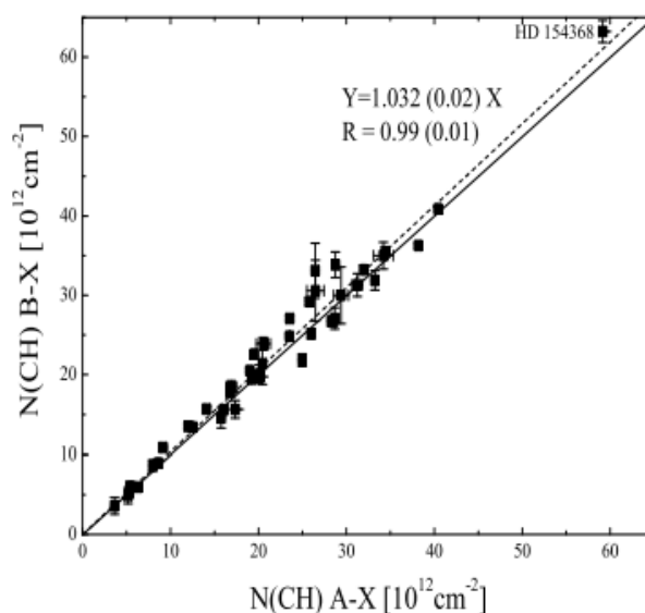
Рисунок 3.15. Сравнение лучевой концентрации, вычисленной для полос B-X (0, 0) и (1, 0) межзвездной молекулы CH. Отметим, что данные для двух пекулярных объектов (HD34078 и HD147889) не представлены на графике.
