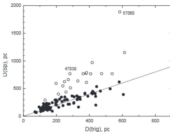
Рисунок 4.9. Сравнение спектрофотометрических расстояний с тригонометрическими. Выбросы (выделенные жирным шрифтом в таблице 40) показаны незакрашенными кружками. Те же символы используются на последующих графиках. Показана линия одинаковых расстояний.
