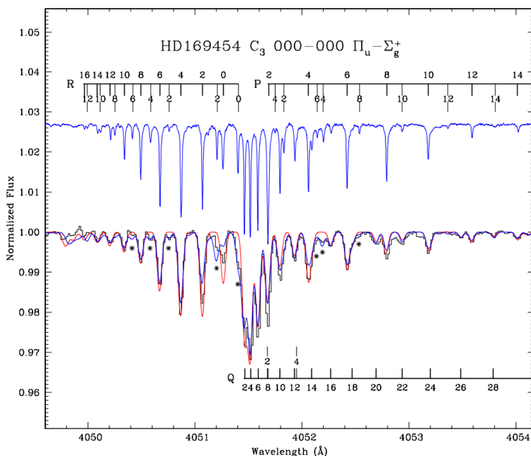
Рисунок 3.2. Спектр полосы C_3 \tilde{A}^1\Pi_u - \tilde{X}^1\Sigma_g^+ 000-000 . Верхний спектр: лабораторный спектр, полученный методом лазерной спектроскопии внутрирезонаторного затухания (cavity ring-down spectroscopy) в плоской плазменной струе. Нижний спектр: астрономический спектр HD 169454 (черный). Положения линий вращения отмечены толстыми линиями. Тонкие линии отмечают вращательные переходы, возникающие из-за возмущающих состояний на основе анализа Zhang et al. (2005). На астрономический спектр наложены аппроксимирующие кривые: красная кривая представляет собой синтетический спектр с использованием только невозмущенных линий; синяя кривая - линии возмущенных переходов включены в аппроксимацию. Обратите внимание на расхождение наблюдений и синтетических спектров в случае линии R(0) (см. текст).
