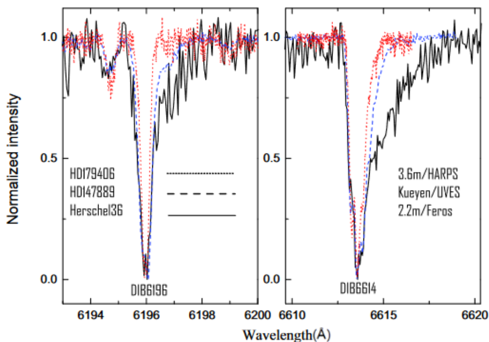
Рисунок 5.64. Развитие красного крыла в профиле с увеличением ротационной температуры некоторых молекул, например, C_2 (Krełowski et al. 2016a).
