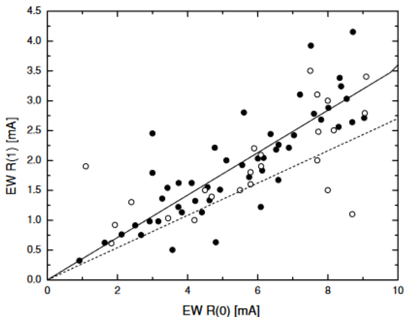
Рисунок 3.23. Соотношение эквивалентных ширин линий CN R(0) и R(1) . Наши измерения отмечены черными кружками, а литературные данные — светлыми кружками. Пунктирная линия представляет отношение эквивалентных ширин для T = 2.725 K. Сплошная линия — линейная аппроксимация представленных данных соответствует T = 3.18 K.
