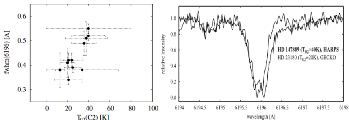
Рисунок 5.31. (Слева) Ширина профиля ДМП 6196 зависит от температуры возбуждения T_{02} молекулы C_2 ; (Справа) Нормализованные по интенсивности (для наглядности) профили ДМП 6196 Å в спектрах двух объектов с разной температурой вращения.
