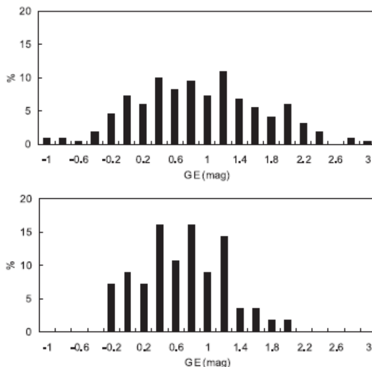
Рисунок 4.6. Процентное распределение эффекта GE для 220 карликов O-B3 на расстоянии до 400 пк (верхний график) и суб-выборка тех же звезд с ошибками параллакса менее 15 процентов (нижний график).
