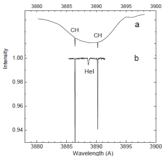
Рисунок 2.29. Широкий профиль звездной линии водорода в спектре \zeta Oph и узкие межзвездные линии «до» (a) и «после» (b) нормализации на профиль звездной линии.
