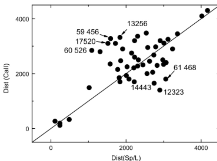
Рисунок 2.26. Сравнение расстояний, полученных методом спектрального параллакса и Ca II-методом.
