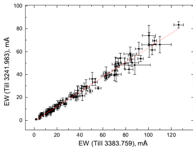
Рисунок 2.12. Сравнение эквивалентной ширины двух межзвездных линий ионизированного титана.
