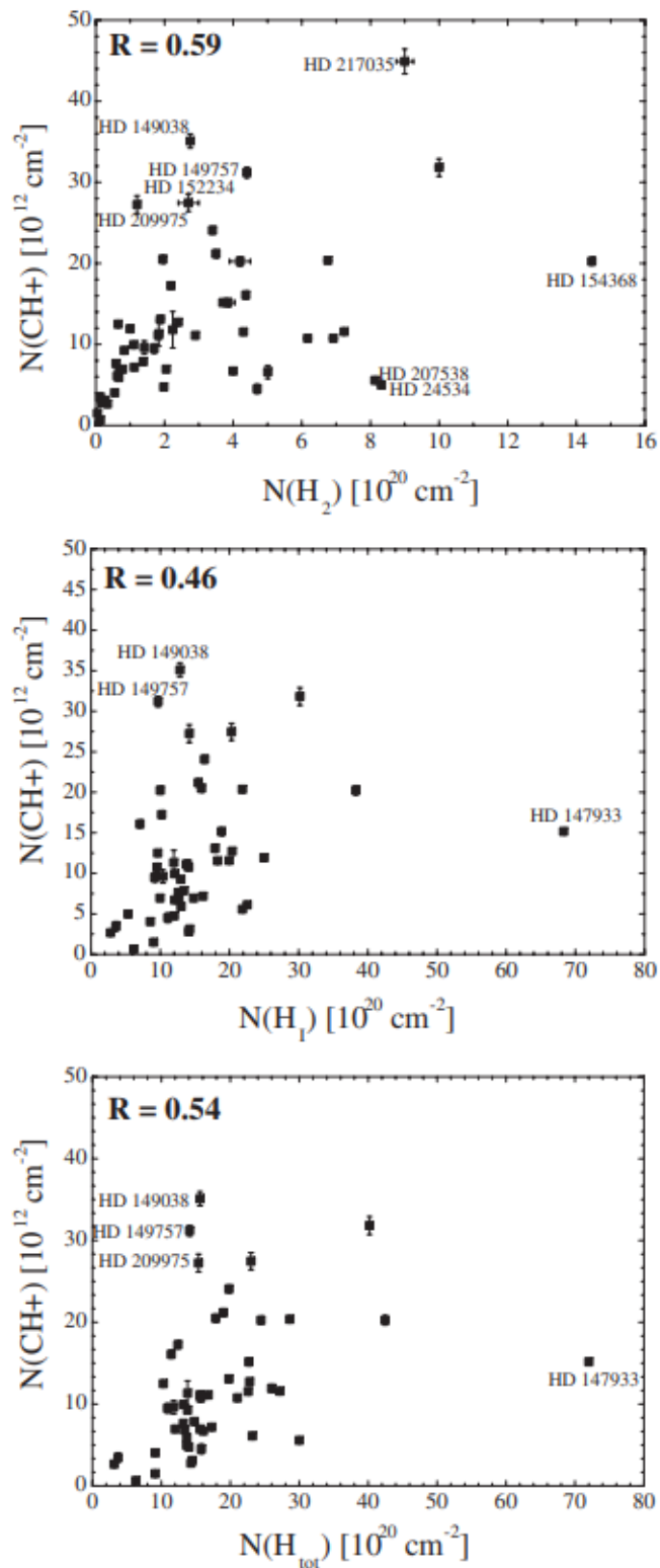
Рисунок 3.16. Сравнение лучевых концентраций молекулы \text{CH}^+ и \text{H}_2 (вверху), \text{H I} (в середине) и \text{H}_{\text{tot}} – внизу. Коэффициент корреляции, равный 0.59, 0.46, 0.54 соответственно свидетельствует об отсутствии линейной связи между этими парами компонент МЗС.
