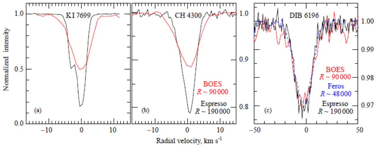
Рисунок 1.11. Сравнение профилей межзвездных линий в спектре HD23180, полученные на разных инструментах с разным спектральным разрешением.
