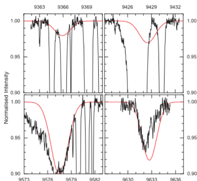
Рисунок 5.81. То же самое, что на рисунке 5.80, но для HD183143.
