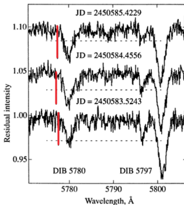
Рисунок 5.35. Изменение интенсивности диффузной полосы 5797 с фазой. Вертикальная красная линия слева от ДМП 5780Å имеет одинаковую высоту для всех трех фаз и служит для сравнения. Глубина ДМП 5797 на нижнем спектре в \sim 2 раза больше, чем на верхнем.
