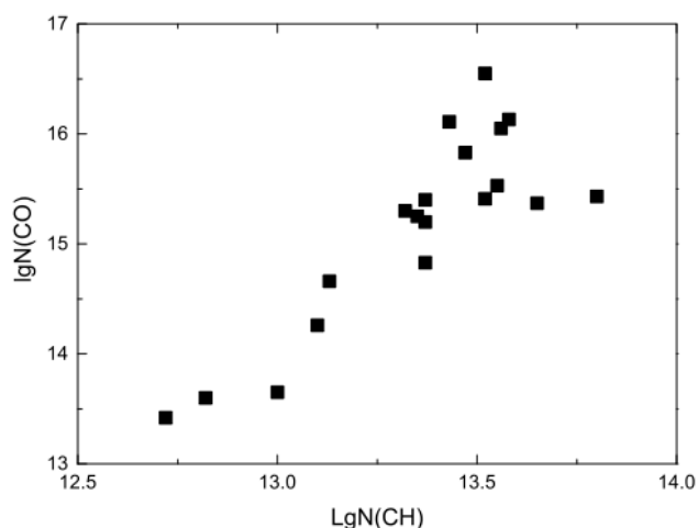
Рисунок 2.18. Позитивная корреляция между лучевыми концентрациями межзвездных молекул CH и CO.
