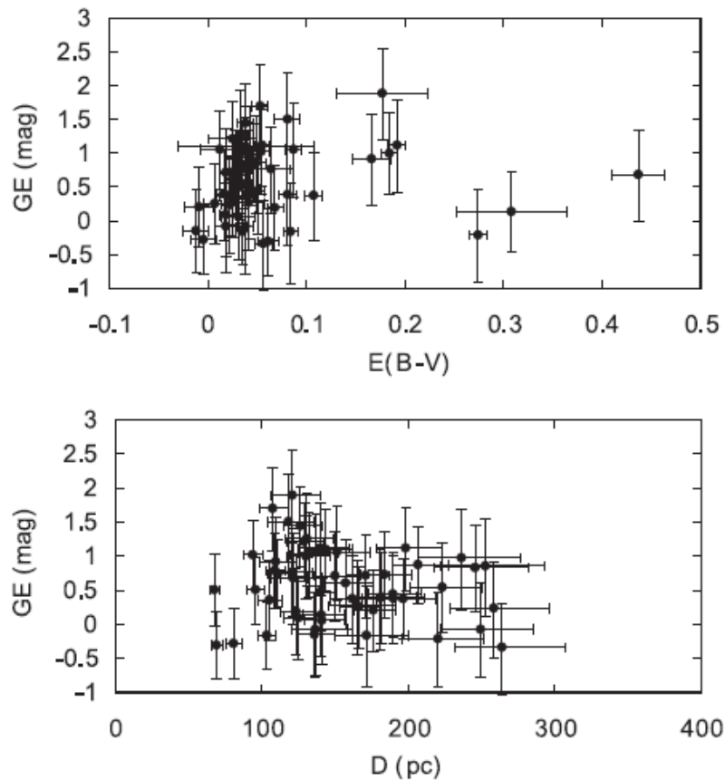
Рисунок 4.2 Эффект GE в зависимости от E(B - V) и расстояний Hipparcos для звезд с ошибкой параллакса, не превышающей 15 %.
