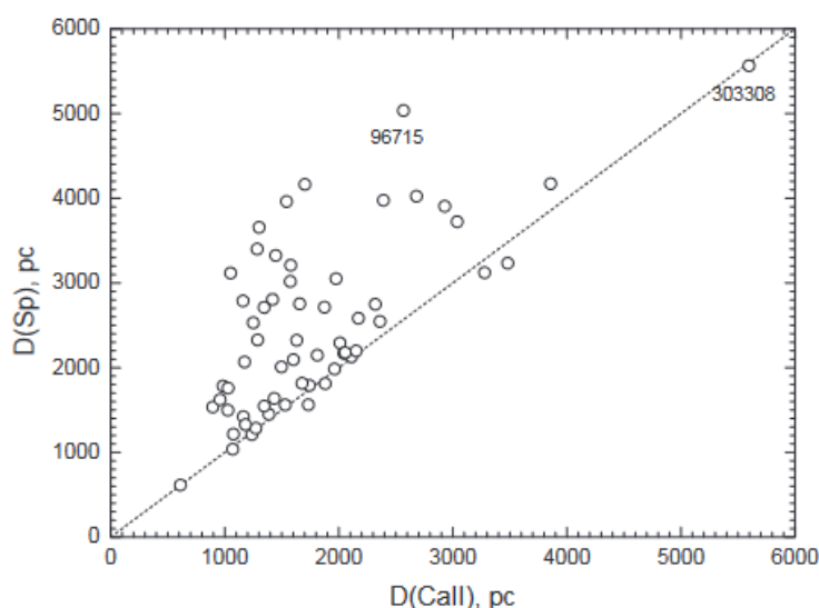
Рисунок 4.12. Сравнение Ca II и спектрофотометрических расстояний для «далеких» объектов из таблицы 41.
