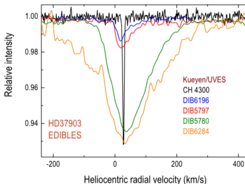
Рисунок 5.46. Широкие и узкие ДМП в гелиоцентрической шкале лучевых скоростей в спектре HD 37903.
