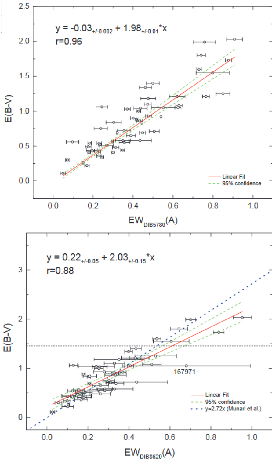
Рисунок 5.22. EW_{5780} и EW_{8620} как индикаторы E(B-V) . Наблюдаемый разброс, не связан с ошибками измерений. Горизонтальная пунктирная линия на нижнем графике указывает верхний предел E(B-V) выборки Munari et al. (2008), чье уравнение связи также показано. Примечание: выборки не идентичны.
