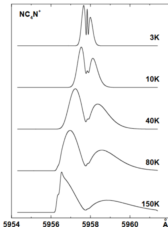
Рисунок 5.53. Изменение профиля молекулы \text{NC}_4\text{N}^+ с температурой. При моделировании использовалось разрешение 50000.
