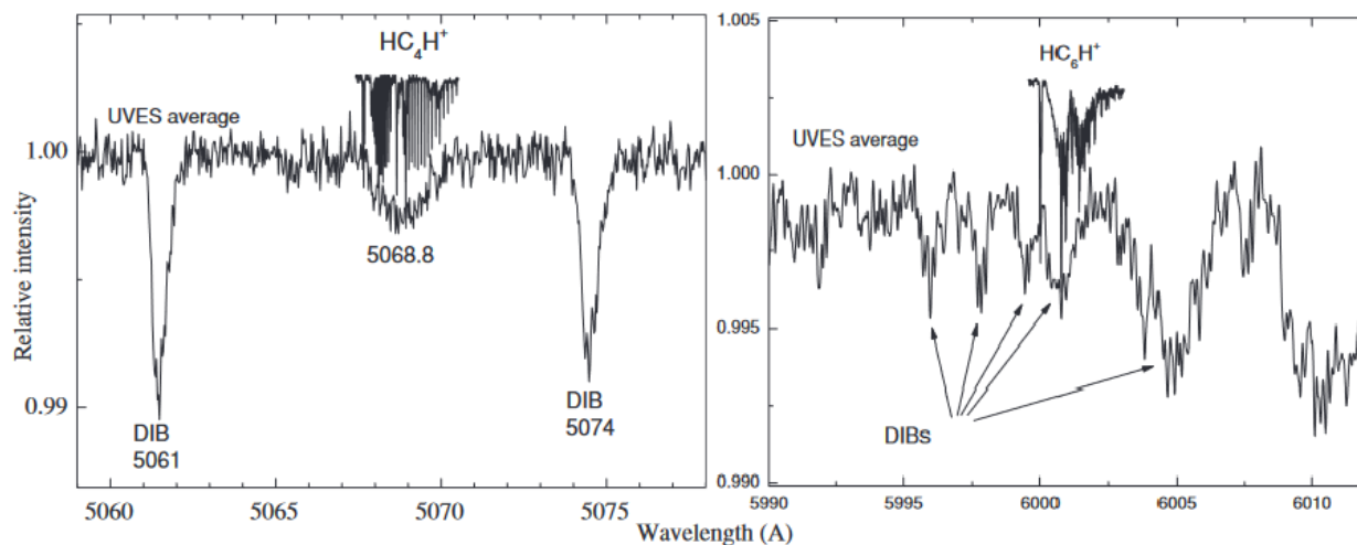
Рисунок 5.54. Сравнение лабораторных спектров молекул \text{HC}_4\text{H}^+ и \text{HC}_6\text{H}^+ (Motylewski et al. 2000) с усредненным спектром 11 покрасневших звезд ( S/N \sim 2000 ).
