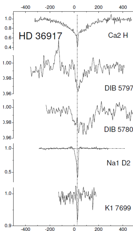
Рисунок 5.40. Красное смещение ДМП 5780. Подобный эффект также наблюдается у некоторых звезд из ассоциации Ori OB1 (Krelowski et al, 2015).
