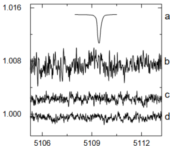
Рисунок 3.33. Область длин волн линии 5109 молекулы C_5 , представленная профилем Гаусса (a). (b) - усредненный спектр 32-х объектов ( R = 120\,000 ) из Терскола. (c) - усредненный спектр ESO CES 3-х объектов типа \zeta (HD 148184, 149757, 179406); (d) - усредненный спектр ESO CES 4-х объектов типа \sigma (HD 143275, 144217, 144470, 147165).
