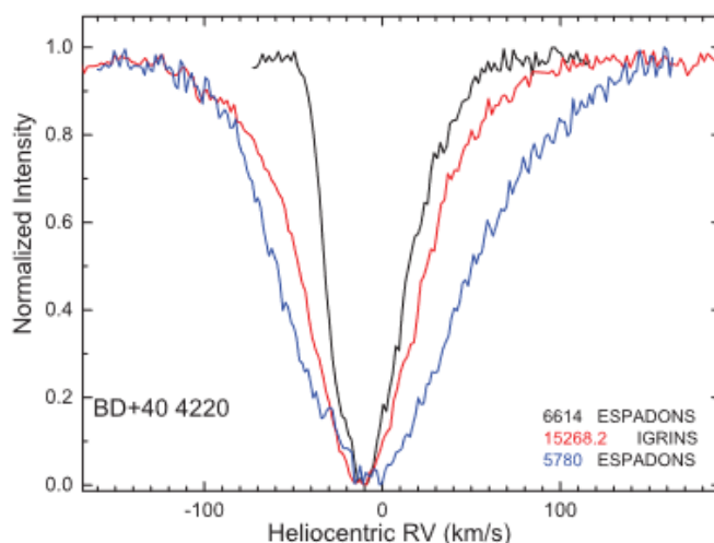
Рисунок 5.4. Сравнение профилей двух известных ДМП 5780 Å (синий) и 6614 Å (черный) с инфракрасной ДМП 15268 Å (красный) в шкале лучевых скоростей. Профиль ДМП 15268 Å почти идеально симметричен в отличие от ДМП из видимой области спектра.
