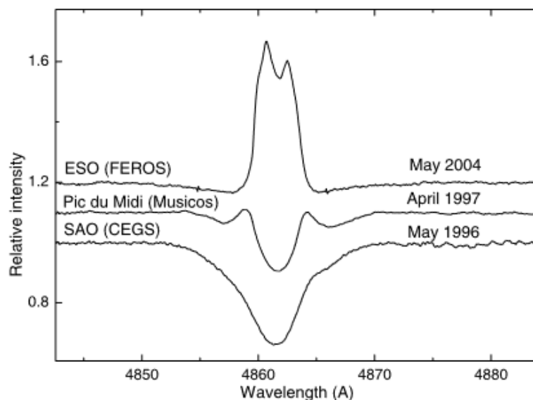
Рисунок 5.41. Переменность профиля линии H \beta в спектрах звезды HD143275.
