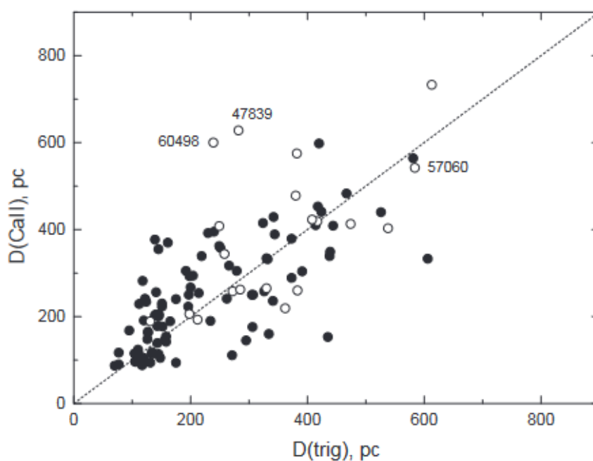
Рисунок 4.11. Сравнение тригонометрических и Ca II расстояний. Светлые кружки соответствуют тем же выбросам, что и на рисунке 4.9. Показана линия равных расстояний Y=X .
