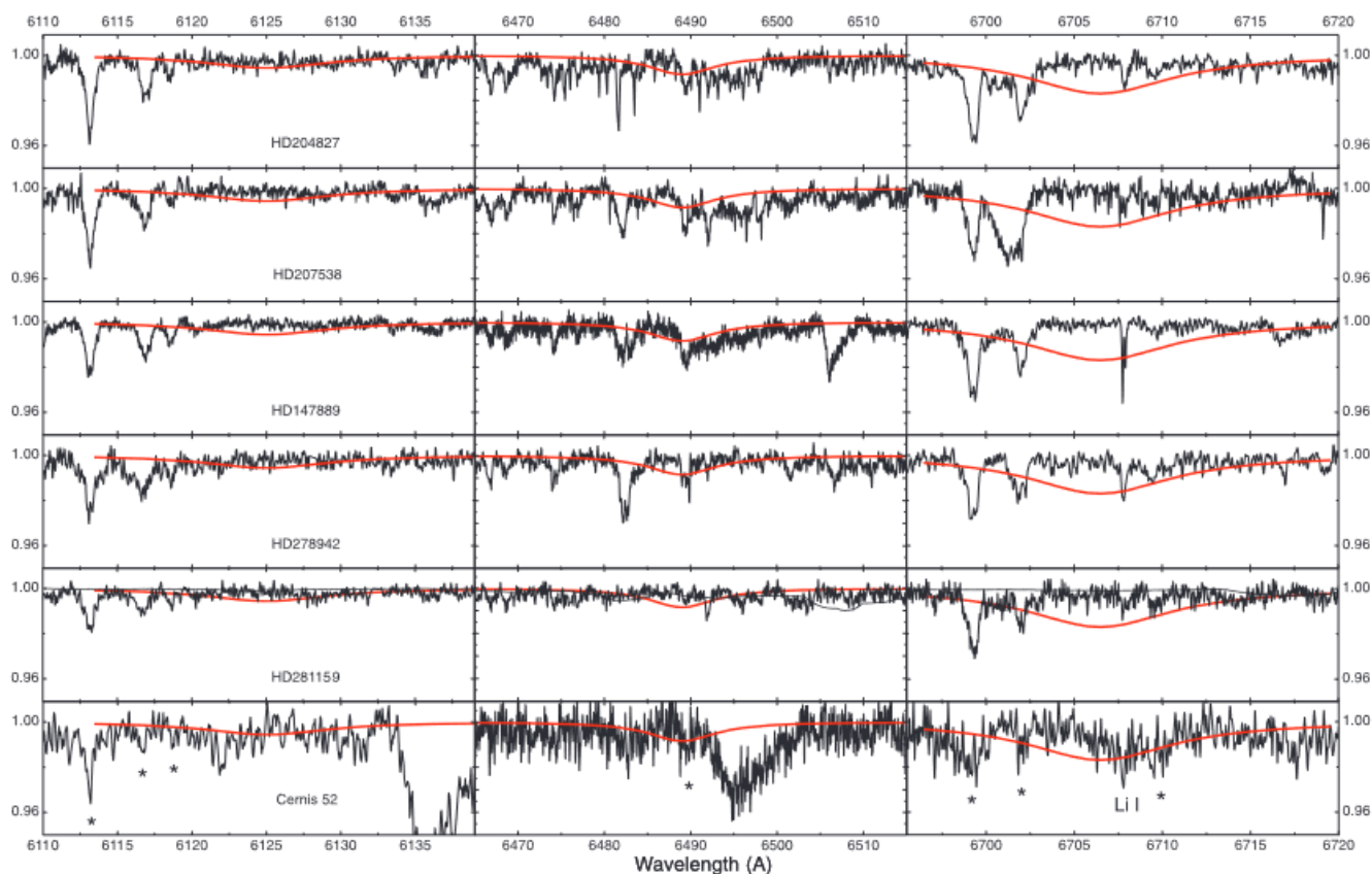
Рисунок 5.61. Спектры звезд программы в области трех основных линий катиона нафталина. Обратите внимание, что вертикальная шкала одинакова на всех графиках: красные профили Лоренца соответствуют ширине и соотношению интенсивностей линий нафталина в лабораторном спектре. Интенсивность самой сильной линии нормализована по глубине абсорбции, видной в спектре Cernis 52 (правый нижний рисунок). Обратите внимание, интенсивность линий растет от синего к красному, например, пик \sim 6125 Å должен быть в три раза слабее самого сильного \sim 6707 Å. Известные ДМП отмечены звездочками; обратите внимание, что те, что в Cernis 52, самые слабые. Черная пунктирная линия, видимая в спектре HD 281159, является синтетическим спектром, рассчитанным с использованием модели атмосферы Kurucz (1993) с T_{\text{eff}} = 15\,400 K, \log g = 3,75 и v \cdot \sin i = 152 км/с, согласно Montesinos et al. (2009).
