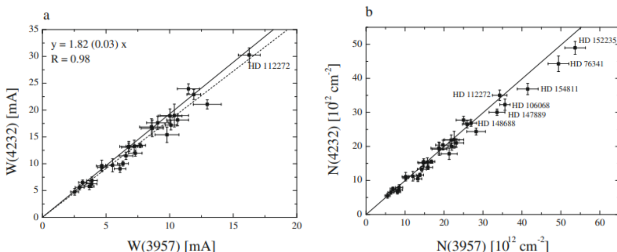
Рисунок 3.18. а) Соотношение эквивалентных ширин полос 3957 и 4232. Сплошная линия соответствует отношению эквивалентных ширин, рассчитанному в отсутствии эффектов насыщения с использованием силы осциллятора Larsson & Siegbahn (1983), прерывистая линия представляет линейную аппроксимацию наблюдаемых данных; б) соотношение лучевых концентраций. Сплошная линия представляет равные значения, полученные из обеих полос. На рисунке б доплеровское расщепление, наблюдаемое у HD 112272 и 148688, сдвигает точки в область с меньшим эффектом насыщения.
