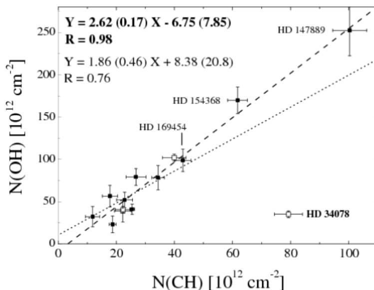
Рисунок 3.12. Сравнение лучевой концентрации молекул OH и CH. Закрашенные точки – наши определения содержания OH, светлые точки – литературные данные. Пунктирной линией представлена зависимость с исключением одной точки данных - HD 34078 (уравнение выделено жирным шрифтом). В этом случае коэффициент корреляции очень высокий и достигает 0.98. В скобках указана ошибка коэффициентов уравнения.
