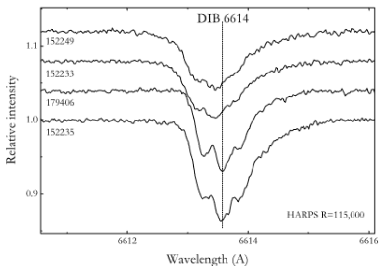
Рисунок 1.9. «Голубой» сдвиг ДМП 6614 в тех же двух объектах ассоциации Sco OB1 что и на рисунке 1.8.
