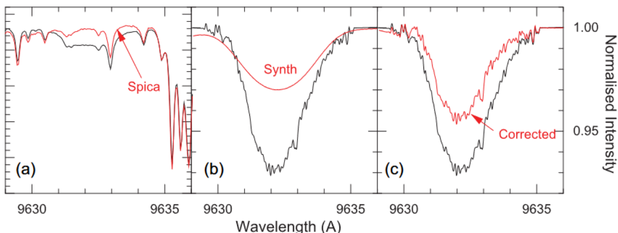
Рисунок 5.79. Последовательные этапы коррекции профиля ДМП 9633 на примере HD80077. (a) Начальный этап: исходный спектр, загрязненный сильными теллурическими линиями, показан вместе со спектром Спика, служащей дивайзером. (b) Профиль ДМП с удаленными теллурическими линиями (черный). Плавная красная кривая - синтетический не-ЛТР профиль звездной линии Mg II 9632 Å, рассчитанный с параметрами, указанными в таблице 70. (c) Заключительный этап: профиль ДМП 9633 после учета линии Mg II показан вместе с неисправленным профилем.
