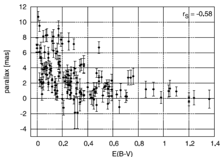
Рисунок 2.4 То же самое, что и на рисунке 2.1, но для межзвездного покраснения.
