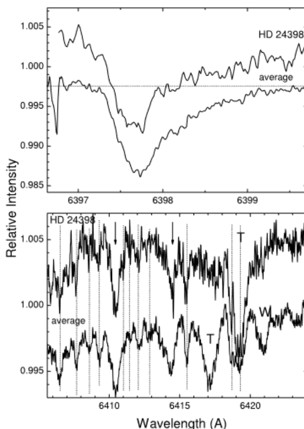
Рисунок 5.19. (Верх) Показан Профиль ДМП 6398 с типичным для многих диффузных полос протяженным красным крылом. (Низ) Пунктирные линии – новые или подтвержденные ДМП с уточненной нами длиной волны из (Galazutdinov et al. 2005a). Стрелками обозначены известные ДМП, указанные в обзоре Galazutdinov et al. (2000a). Вопросительным знаком указаны особенности, которые, вероятно, являются межзвездными, но, по-видимому, блендированные со звездными линиями. Т - ДМП из обзора Tuairisg et al. (2000). Уровень S/N превышает 1000 – см. цену деления вертикальной шкалы.
