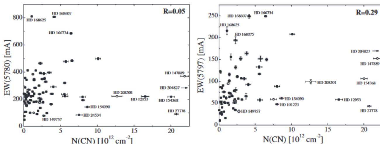
Рисунок 5.27. Отсутствие связи между лучевой концентрацией CN и эквивалентными ширинами главных ДМП (Weselak et al. 2008b).
