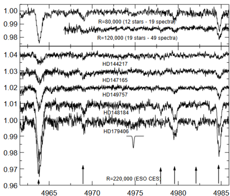
Рисунок 3.32. Верхний график: уже опубликованный (Galazutdinov et al. 2001) усредненный спектр R = 80000 в сравнении с усредненным спектром R = 120000 , полученный нами на обсерватории Терскол. Нижний график: отдельные спектры ESO спектрографа CES ( R=220000 ) и профиль гаусса, представляющий линию C_5 4975 \text{ \AA} . Стрелки указывают на диффузные межзвездные полосы.
