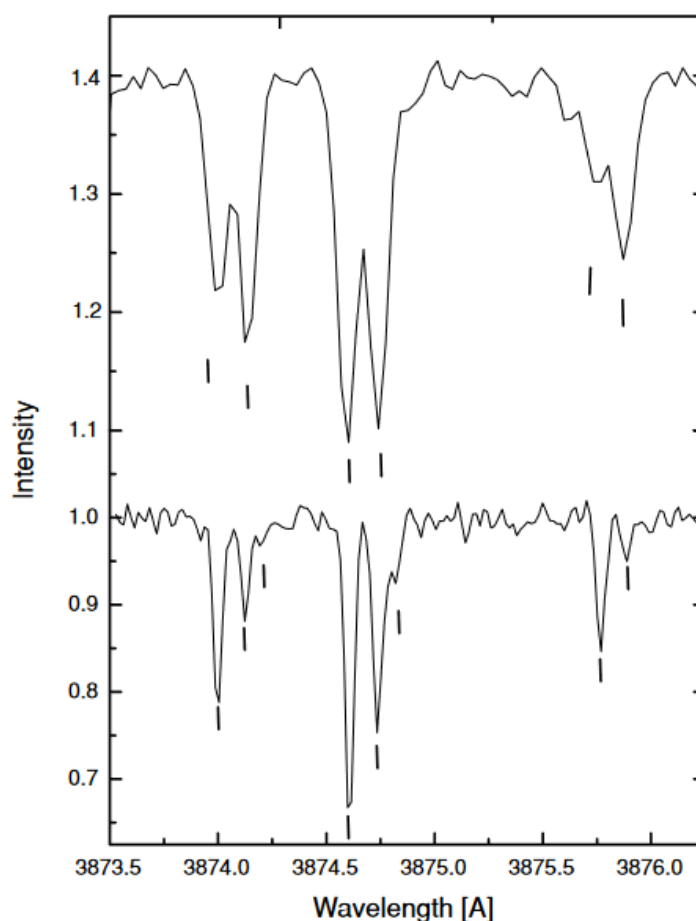
Рисунок 3.22. Линии полосы B^2\Sigma^+ - X^2\Sigma^+ (0,0) молекулы CN в направлениях на HD 306097 (верхний спектр) и BD-14°5037 (нижний спектр), полученные с помощью спектрографов FEROS и UVES соответственно. Видимое расщепление компонентов очень редко встречается в линиях CN. Обратите внимание на эффекты насыщения в доминирующем доплеровском компоненте линии R(0) в BD-14°5037 и очевидно разные отношения интенсивностей R(0)/R(1) в отдельных доплеровских компонентах в HD 306097, что указывает на разные вращательные температуры в двух облака в направлении на этот объект.
