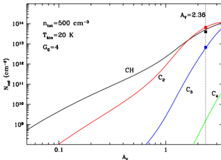
Рисунок 3.7. Содержание молекул CH, C_2 , C_3 и C_4 в зависимости от общего поглощения A_V согласно модельным расчетам.
