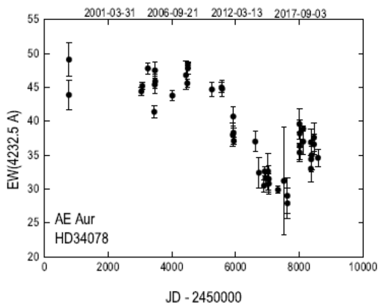
Рисунок 5.43. Интенсивность линии \text{CH}^+ 4232 Å за период с 1997 по 2019 год. За падением EW в 2010–2015 годах, последовал рост в 2016–2019 годах.
