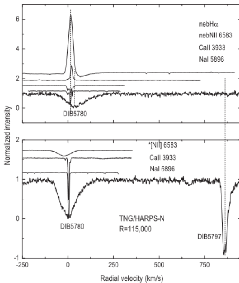
Рисунок 5.47. Верх. ДМП 5780 в спектре HD 37022 в шкале лучевых скоростей вместе с другими межзвездными и небулярными линиями. Шкала ординат произвольна. Две пунктирные линии отмечают положение нулевого компонента скорости и положение пика ДМП 5780, явно смещенного в красную сторону на \sim 30 км/с. Низ. То же самое для «обычного» облака в спектре HD 24398. Этот объект не имеет небулярных линий. ДМП 5780 не смещен.
