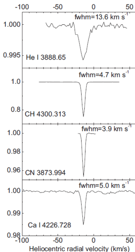
Рисунок 2.30. Сравнение профилей межзвездных линий в спектре ζ Oph: видно, что линия He I* 3889 наиболее широкая.
