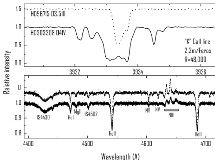
Рисунок 4.13. Сравнение спектров двух звезд, отмеченных на рисунке 4.12. Обратите внимание на близкое сходство Sp/L и диффузных полос на 4430Å. Сложный профиль линии CaII К в спектре более далекого объекта HD 303308 демонстрирует множество отдельных компонентов в отличие от относительно простого профиля CaII в спектре более близкого объекта HD 96715.
