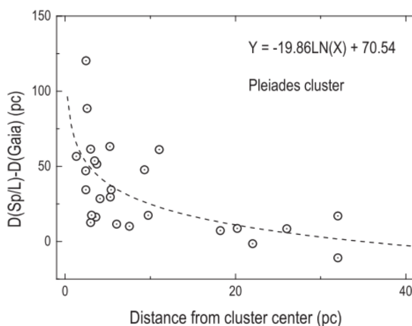
Рисунок 2.36. Зависимость эффекта «серого» межзвездного поглощения от расстояния до центра скопления.
