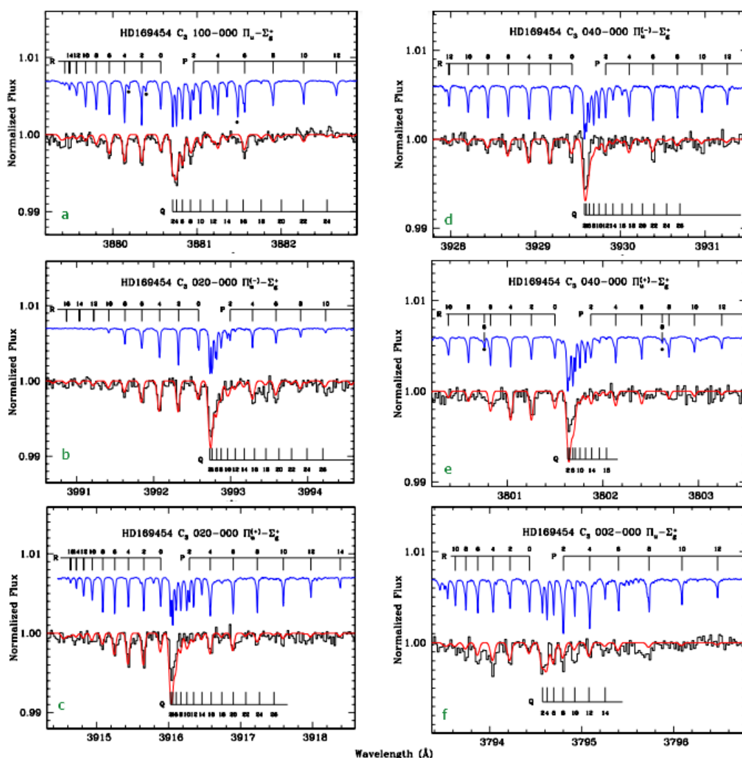
Рисунок 3.3. а) Лабораторный спектр (синяя линия) и астрономический спектр HD 169454 (черный) для полосы C_3 \tilde{A}^1\Pi_u - \tilde{X}^1\Sigma_g^+ 100-000 . Синтетический спектр показан красным цветом. Возмущенные линии отмечены звездочкой; б) Тоже самое для полосы 02^0-000 ; в) Тоже самое для полосы 02^+0-000 ; д) Тоже самое для полосы 04^0-000 ; е) Тоже самое для полосы 04^+0-000 ; д) Тоже самое для полосы 002-000 .
