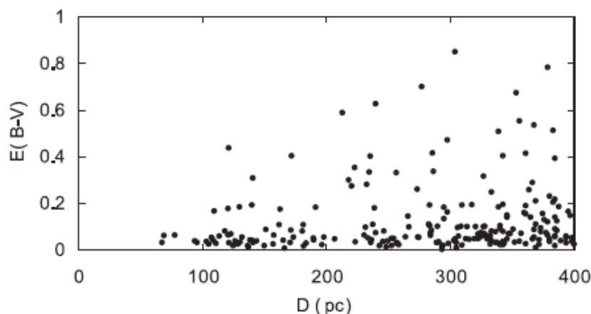
Рисунок 4.3 Зависимость межзвездного покраснения от расстояния.
