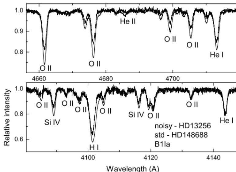
Рисунок 2.27. — Сравнение спектров HD13256 (спектр с более низким S/N) и HD148688 (стандарт B1Ia).
