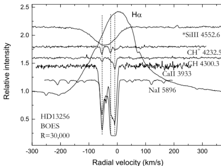
Рисунок 2.17. Компоненты профиля межзвездных линий в шкале лучевых скоростей в направлении HD13256 и профили линий водорода и дважды ионизованного кремния этой звезды.
