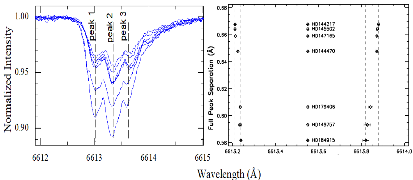
Рисунок 5.66. Положение пиков в профилях очень высокого ( R = 220000 ) разрешения ДМП 6614 (Galazutdinov et al. 2002b, Cami et al. 2004).
