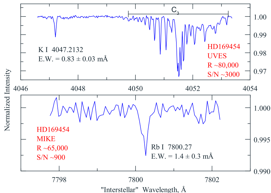
Рисунок 1.1. Примеры профилей слабых межзвездных линий в спектрах с высоким спектральным разрешением и очень высоким соотношением S/N.
