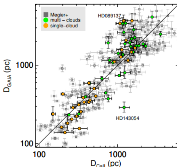
Рисунок 2.9. Связь между оценками расстояния с использованием параллакса GAIA (Bailer-Jones et al. 2018), и дублета Ca II H, K по Megier et al. (2009). Показаны объекты без видимого доплеровского расщепления (оранжевые кружки) и с несколькими компонентами (зеленые кружки) из работы Siebenmorgen et al. (2000).
