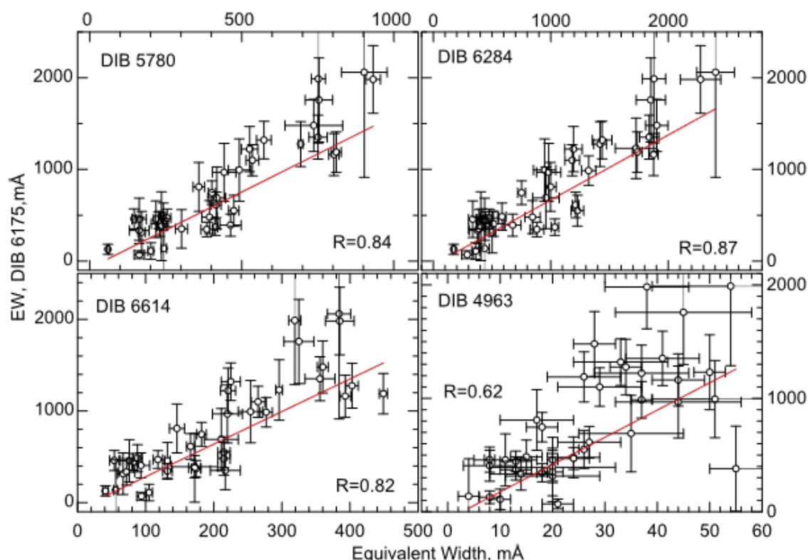
Рисунок 5.12. Корреляция широкой ДМП 6175 с другими, более узкими диффузными полосами. Вероятно, можно утверждать об общей локализации носителей широкой ДМП 6175 и гораздо более узких 5780 и 6284.
