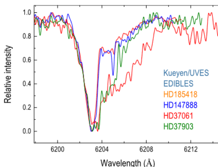
Рисунок 5.45. Профили ДМП 6203 нормализованные к одинаковой глубине для наглядности.
