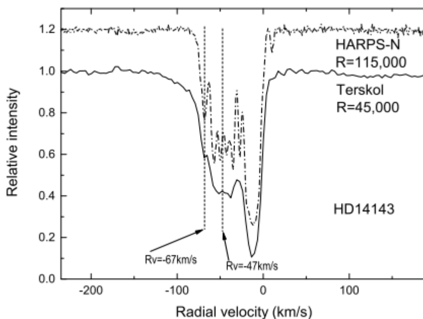
Рисунок 2.24. Увеличение спектрального разрешения позволяет выявить компоненту с наибольшим синим смещением — это приводит к увеличению расхождения между наблюдениями и «плоской» кривой вращения (см. рисунок 2.23). Показаны спектры одного из объектов в направлении l=135^\circ .
