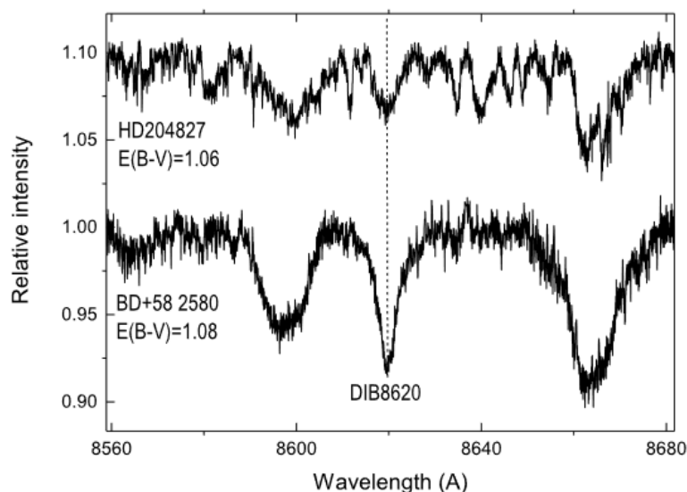
Рисунок 5.23. Спектры двух звезд с одинаковым покраснением E(B-V) .
