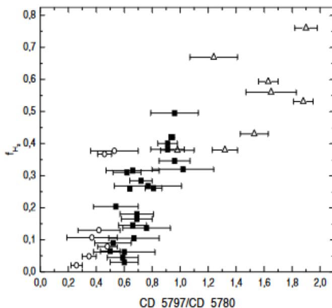
Рисунок 5.26. Корреляции между молекулярной фракцией водорода и отношением интенсивностей диффузных полос 5797 и 5780. Коэффициент корреляции равен 0.83. Объекты типа \sigma обозначены кружками, \zeta — треугольниками. Остальные объекты обозначены черными квадратами (Weselak et al. 2004).
