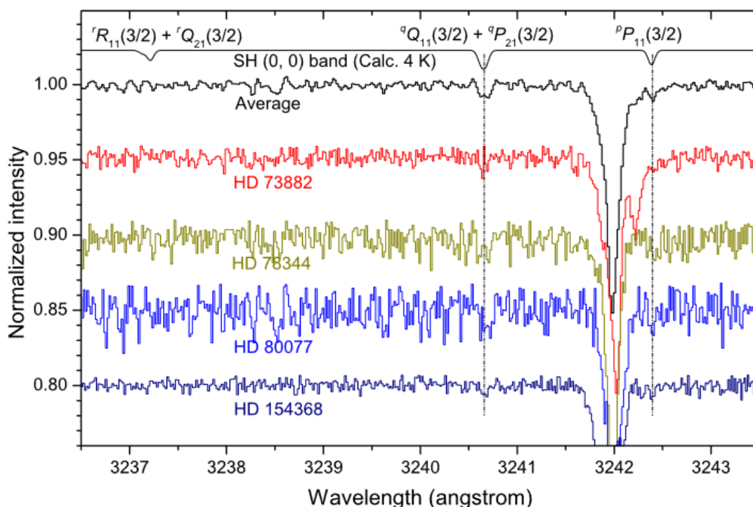
Рисунок 3.31. Спектр полосы SH A 2 Σ + -X 2 Π (0, 0). Сверху вниз: рассчитанный спектр 4 K, усредненный спектр и отдельные спектры в направлении на HD 73882, HD 78344, HD 80077 и HD 154368. Спектры наблюдаемых объектов нормализованы на псевдоконтинуум, т. е. все широкие особенности, включая звездные линии, исключены для наглядности. Длины волн скорректированы в межзвездную шкалу.
