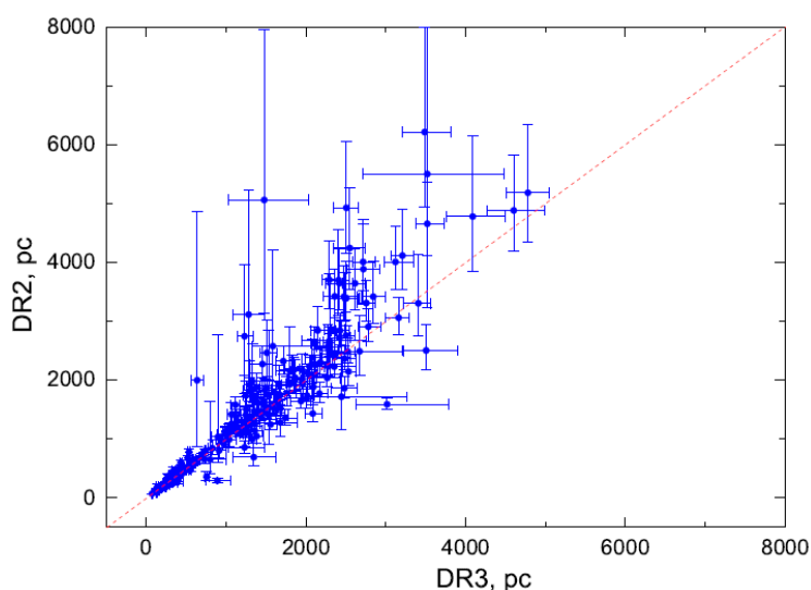
Рисунок 2.13. Сравнение расстояний по данным GAIA DR2 и DR3 для объектов из таблицы 2. Красная пунктирная линия y = x приведена для наглядности.
