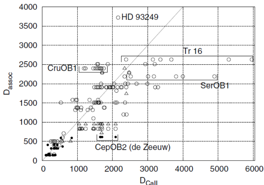
Рисунок 2.7. Расстояния, оцененные по линиям Ca II (абсцисса) в сравнении с расстояниями до ассоциаций из разных источников (ордината). Символы: незакрашенные круги – Humphreys (1978); незакрашенные треугольники – Garmany & Stencel (1992); закрашенные круги – de Zeeuw et al. (1999).
