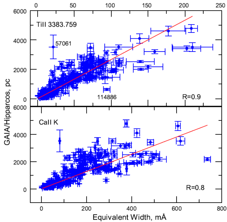
Рисунок 2.11 Зависимость между эквивалентными ширинами межзвездных линий Ti II 3383.759 Å (a) и Ca II K (b) и оценками расстояний, найденных с помощью GAIA/Hipparcos. Также показаны коэффициенты корреляции Пирсона R .
