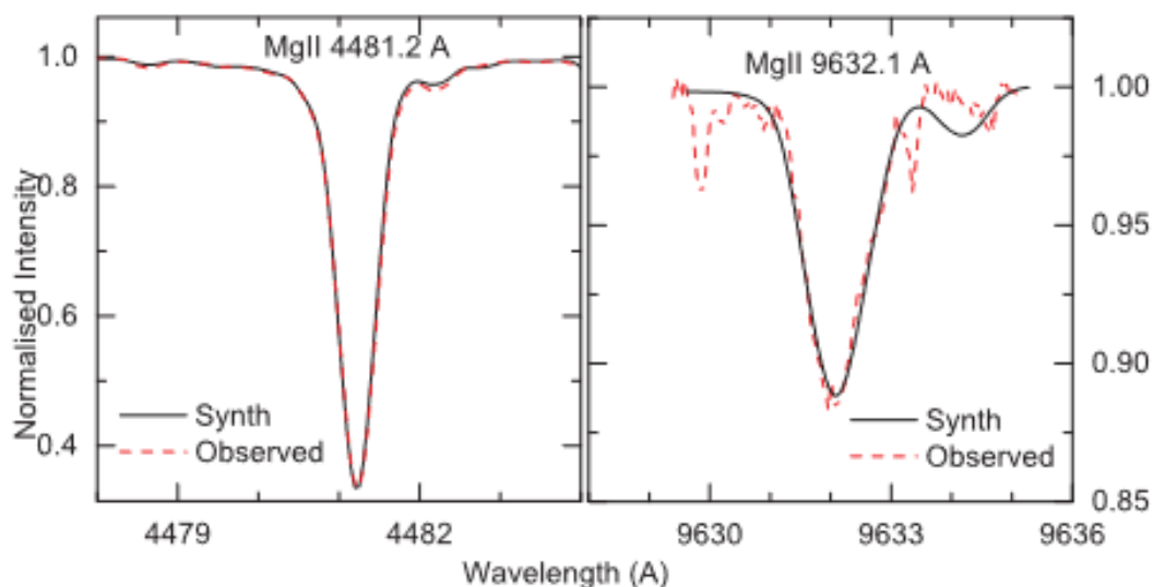
Рисунок 5.78. Профили линий Mg II 4481.2 и 9632.1 Å (красные) в спектре Сириуса, вместе с соответствующим синтетическим спектром (черный). Исправленные силы осцилляторов приведены в таблице 71.
