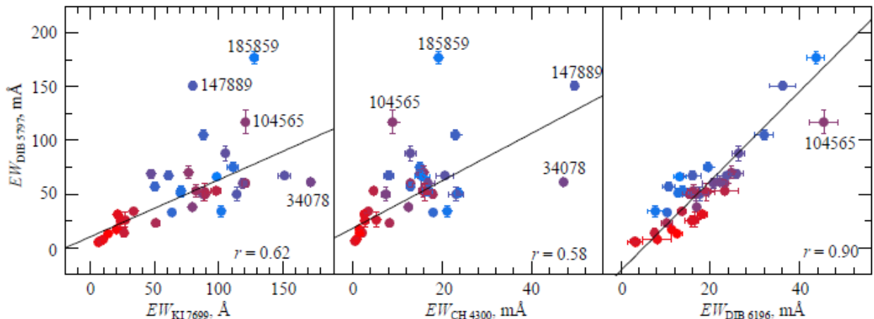
Рисунок 1.12. Корреляция ДМП 5797 и межзвездных СН, К I и ДМП 6196. Коэффициент корреляции указан в каждом случае. Шкала цветов показывает соотношение эквивалентной ширины «главных» диффузных полос 5797/5780 (см. раздел 5.7.3. главы 5).
