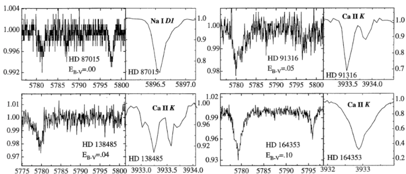
Рисунок 5.24. Диффузные полосы в звездах с небольшим (нулевым) покраснением. В каждом случае наблюдается доплеровское расщепление в атомных межзвездных линиях.
