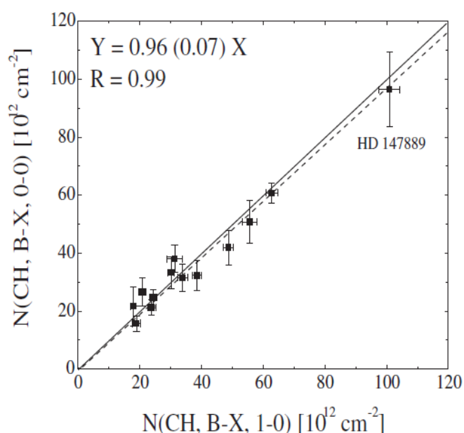
Рисунок 3.14. Сравнение лучевой концентрации, вычисленной для полос В-Х (0, 0) и (1, 0) межзвездной молекулы СН.
