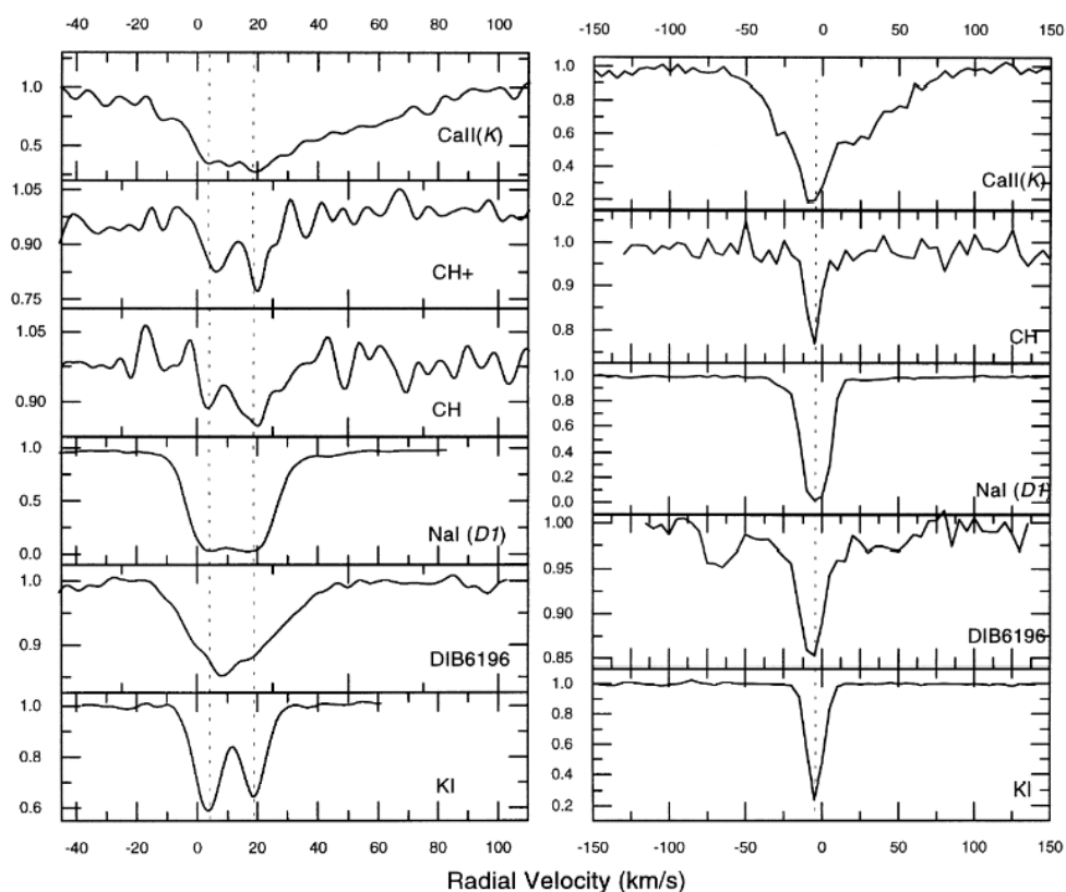
Рисунок 5.1. Профили межзвездных линий в шкале лучевых скоростей HD183143 (слева) и HD186745 (справа) – Galazutdinov et al. (2000). На луче зрения HD183143 наблюдается как минимум два примерно одинаковых облака (см. профили K I и Na I), тогда как в спектре HD 186745 на наблюдается очевидного доплеровского расщепления.
