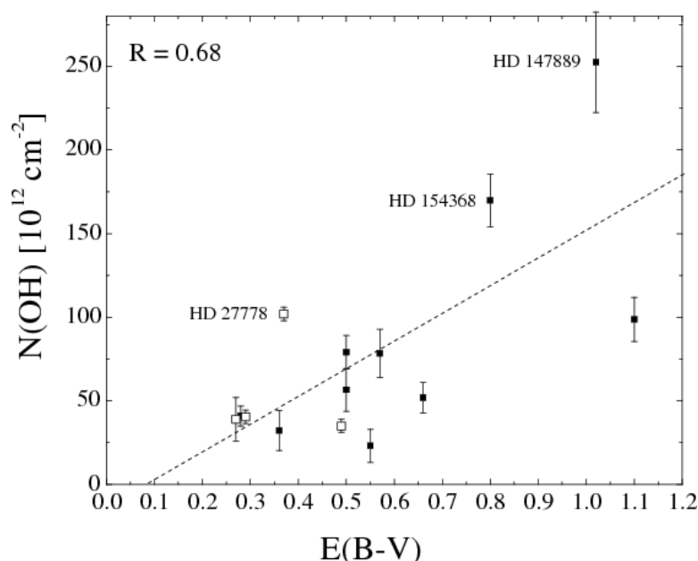
Рисунок 3.11. Связь между лучевой концентрацией молекулы OH и межзвездным покраснением E(B-V) . Молекула OH, вероятно, не наблюдается при E(B-V) ниже 0.08. Светлыми квадратами отмечены объекты с N(OH) из литературы.
