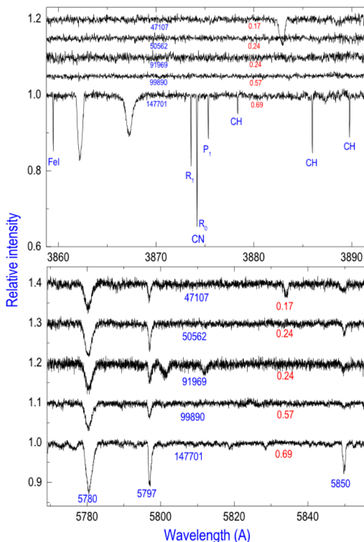
Рисунок 5.28. Покраснение E(B - V) указано красным, под каждым спектром указаны номера HD. (Верх) Сильные молекулярные и атомные межзвездные линии видны только в спектре HD147701; (Низ) «Главные» диффузные полосы 5780 и 5797 Å. Интенсивность обеих ДМП не зависит от покраснения, CH, CN и Fe I.
