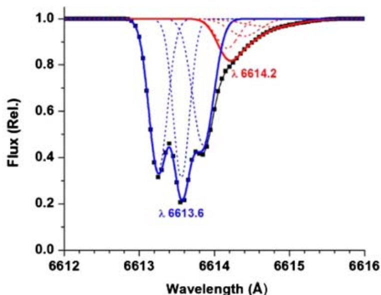
Рисунок 5.67. Деконволюция профиля ДМП 6614 в спектре HD 179406 профилями Гаусса.
