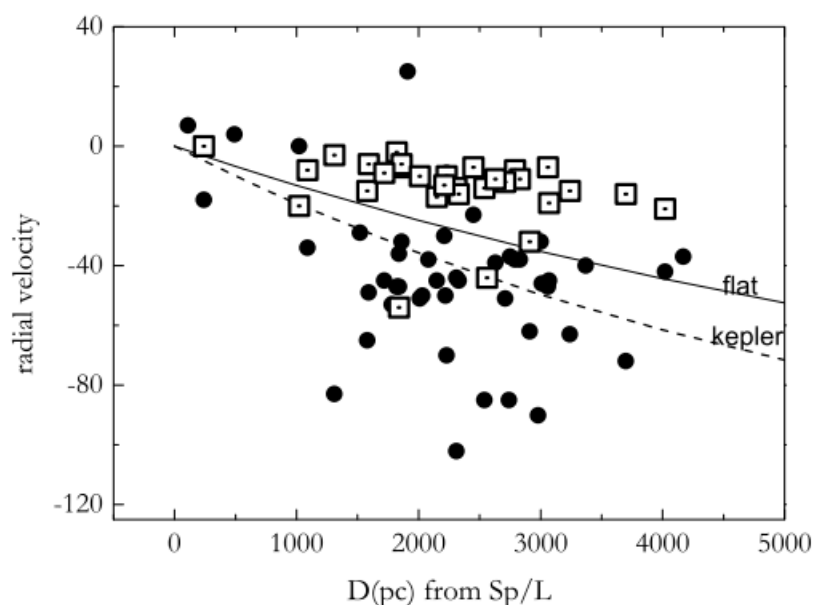
Рисунок 2.28. — Кривые вращения по лучевым скоростям звездных линий (закрашенные кружки) и по линиям межзвездной молекулы CH (квадраты).
