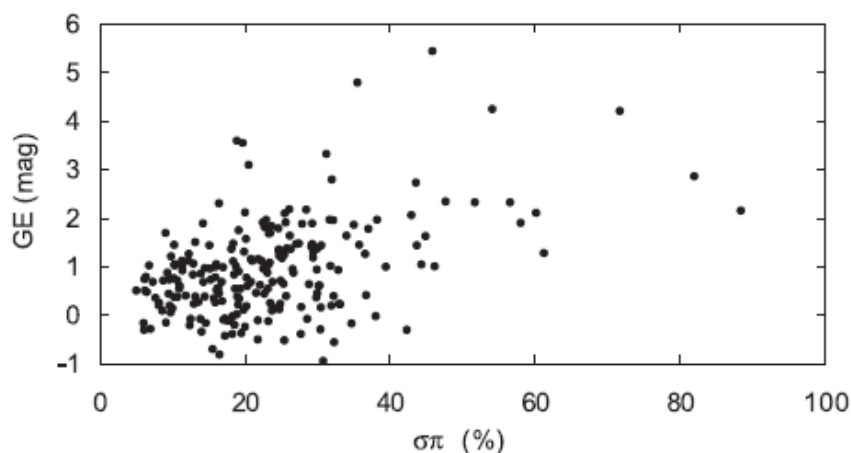
Рисунок 4.4 Зависимость GE от ошибок тригонометрического параллакса Hipparcos.
