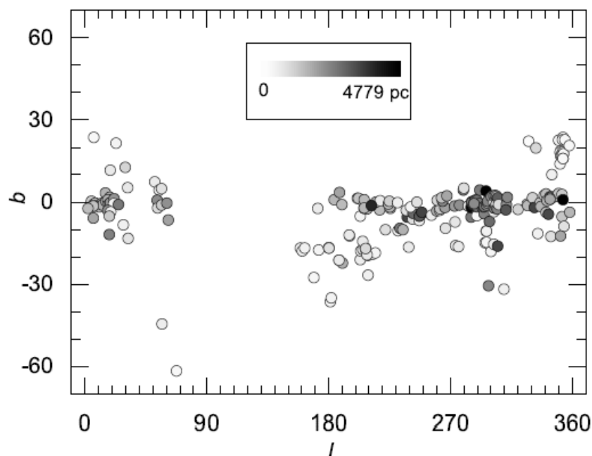
Рисунок 2.10. Местоположение исследуемых объектов в Галактических координатах. Тригонометрическое расстояние показано серой шкалой.
