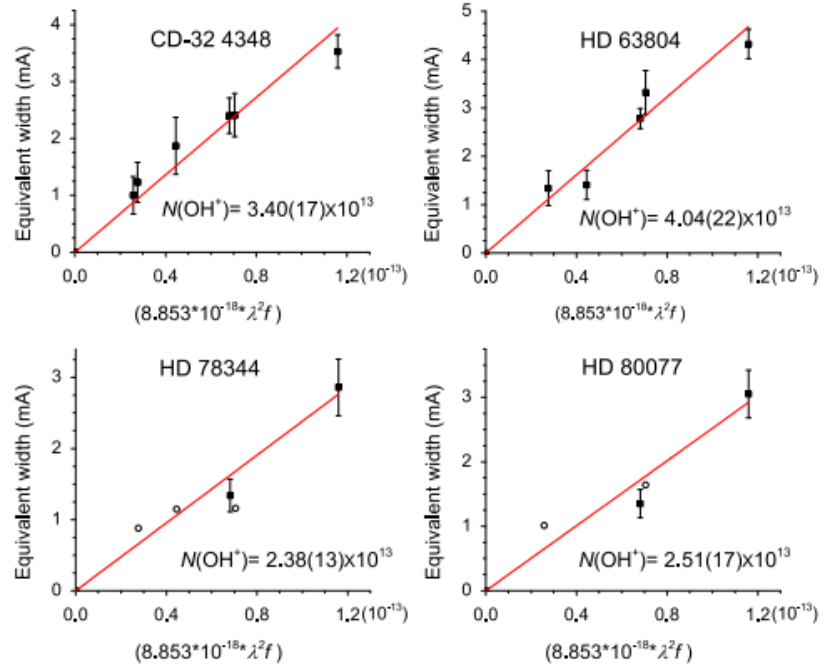
Рисунок 3.10. Взвешенная линейная аппроксимация эквивалентных ширин для определения лучевой концентрации OH + . Незакрашенные кружки означают неуверенное измерение (верхний предел), не включенное в аппроксимацию.
