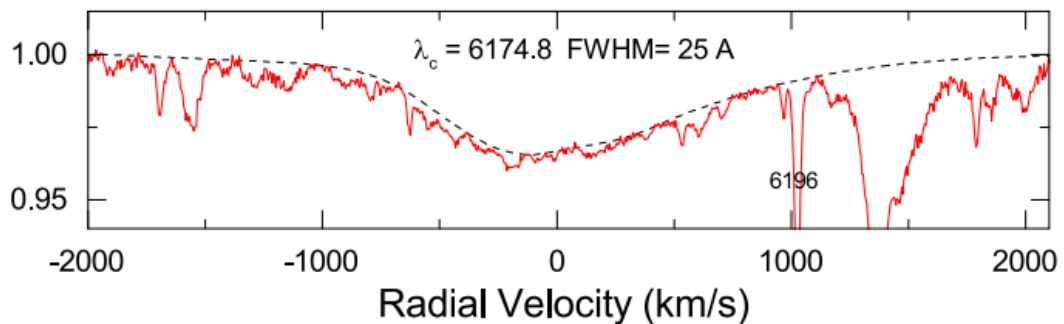
Рисунок 1.5. Профиль широкой диффузной полосы ~6175 асимметричен, блендирован как звездными, так и межзвездными линиями. «Истинный» профиль межзвездной полосы показан прерывистой линией.
