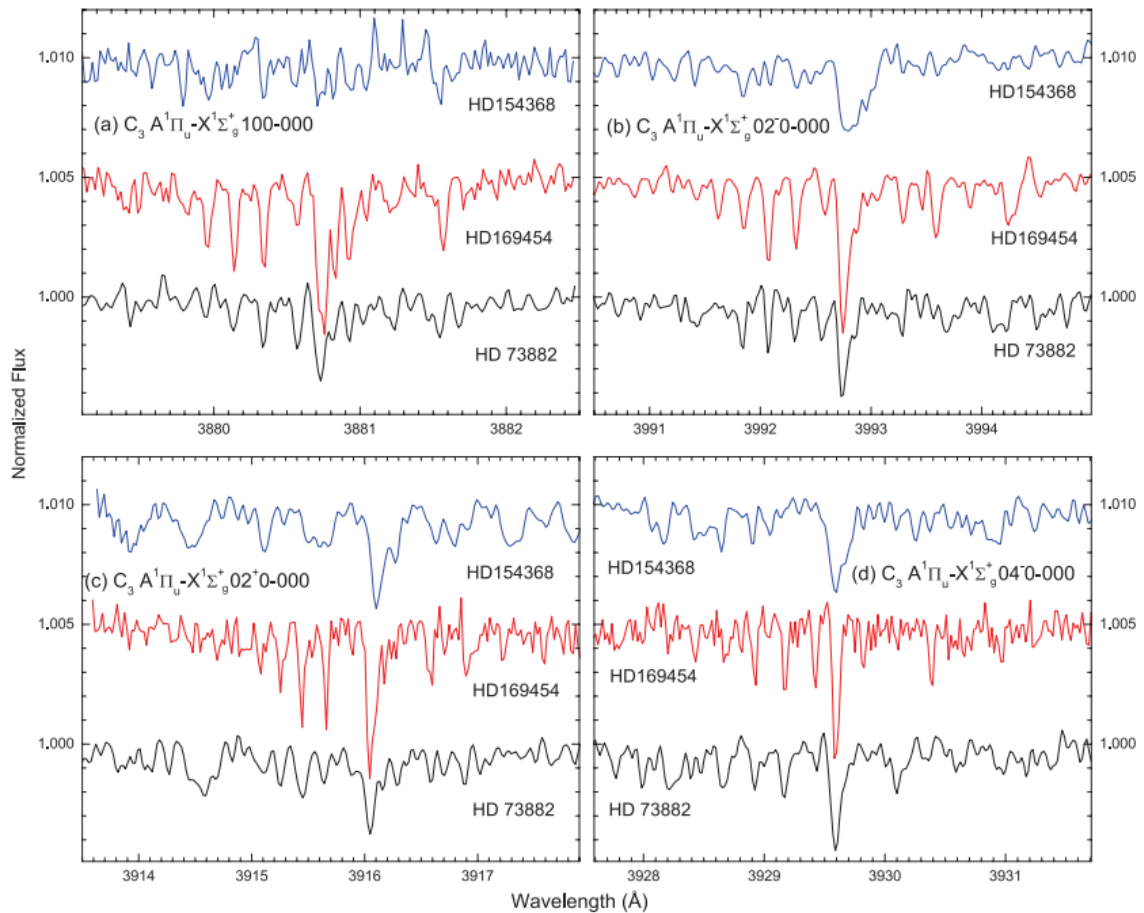
Рисунок 3.1. Четыре колебательные полосы системы \tilde{A}^1\Pi_u - \tilde{X}^1\Sigma_g^+ межзвездной молекулы C_3 в спектрах звезд HD 154368, HD 169454 и HD 73882.
