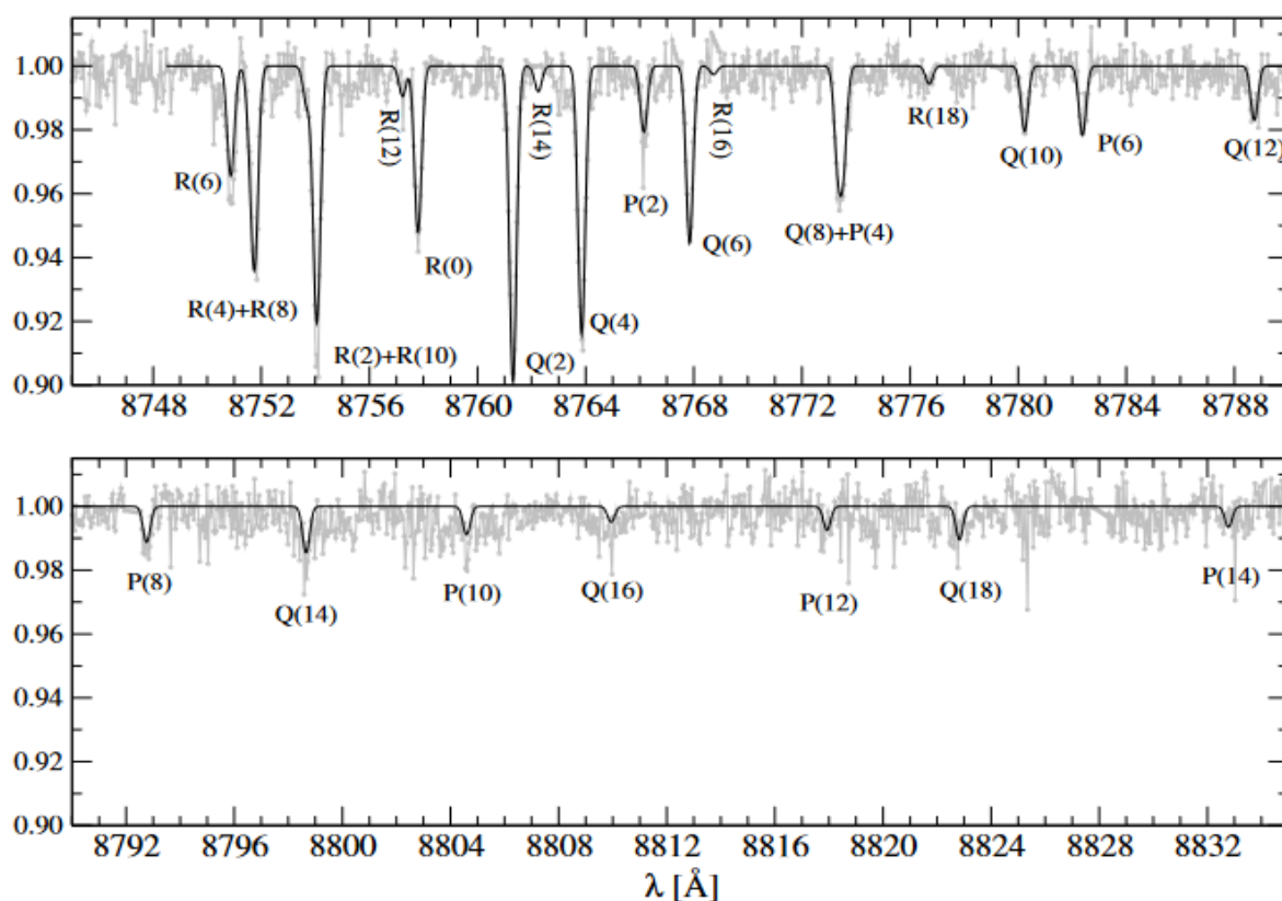
Рисунок 5.29. Аппроксимация профилей линий полосы молекулы C_2 системы Филиппса (2,0) A^1\Pi_u - X^1\Sigma_g^+ в спектре звезды HD204827.
