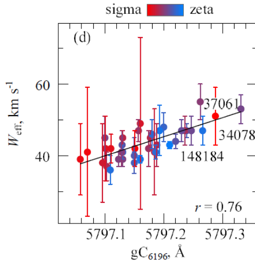
Рисунок 1.13. Зависимость центра тяжести линии от ее эффективной ширины в случае ДМП 5797. Индекс 6196 в подписи оси абсцисс означает, что шкала длин волн опиралась на ДМП 6196.
