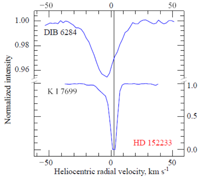
Рисунок 1.10. Различная лучевая скорость межзвездных линий в спектре звезды HD152233, принадлежащей ассоциации Sco OB1. Очевидно, носители ДМП 6284 и атомарный газ занимают разные объемы облака.
