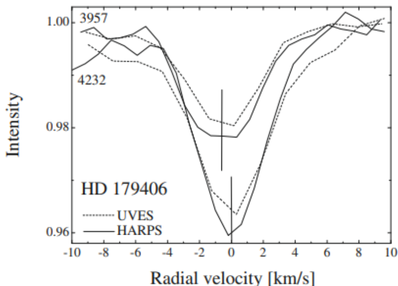
Рисунок 3.19. Систематический сдвиг линии \text{CH}^+ \sim 3957 \text{ \AA} в область более коротких длин волн. Величина сдвига использовалась для коррекции длины волны линии.
