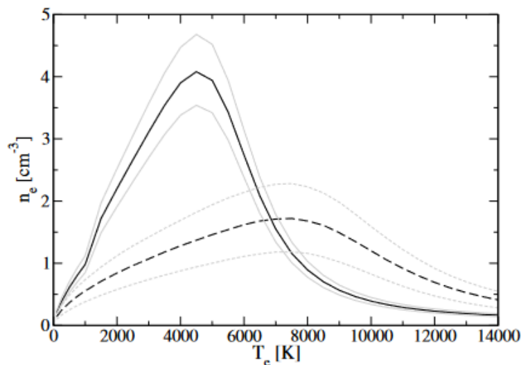
Рисунок 5.32. Кривые n_e(T_e) для MgI/MgII (сплошная линия) и SiI/SiII (пунктирная линия) для облака v = -31 км/с в направлении HD 210839. Точка пересечения этих кривых позволяет определить электронную концентрацию n_e .
