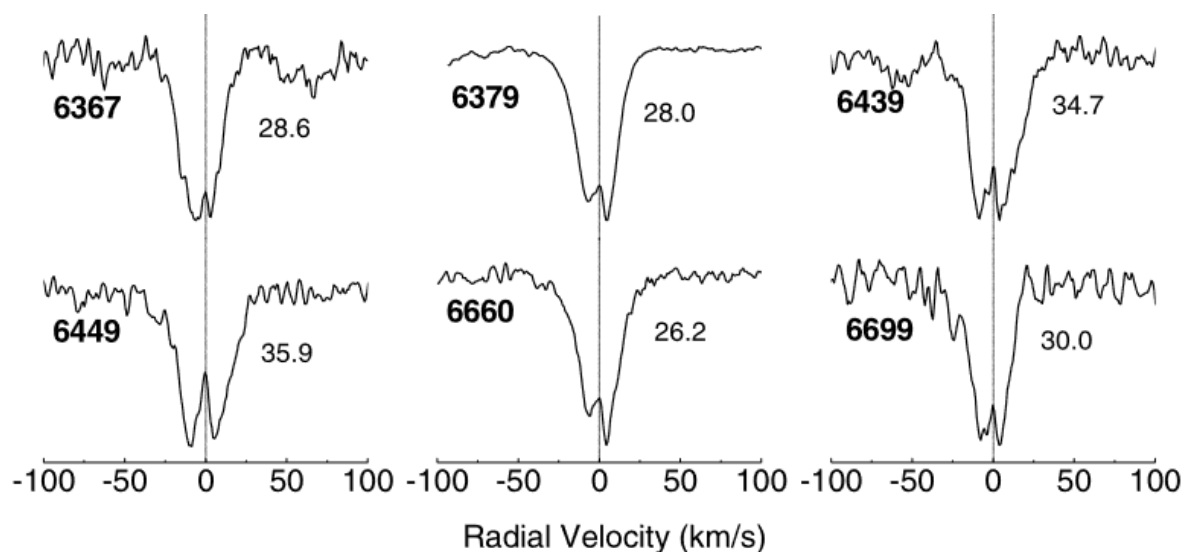
Рисунок 5.20. Нормализованные профили ряда ДМП в спектре HD 147889 шкале лучевых скоростей. Справа указана FWHM каждой ДМП в км/с.
