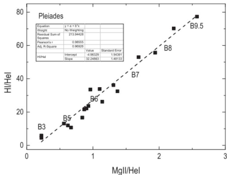
Рисунок 2.34. Отношение интенсивности линий Mg II/He I и He I/H I, служащие для определения спектрального класса по методу Walborn & Fitzpatrick (1990).
