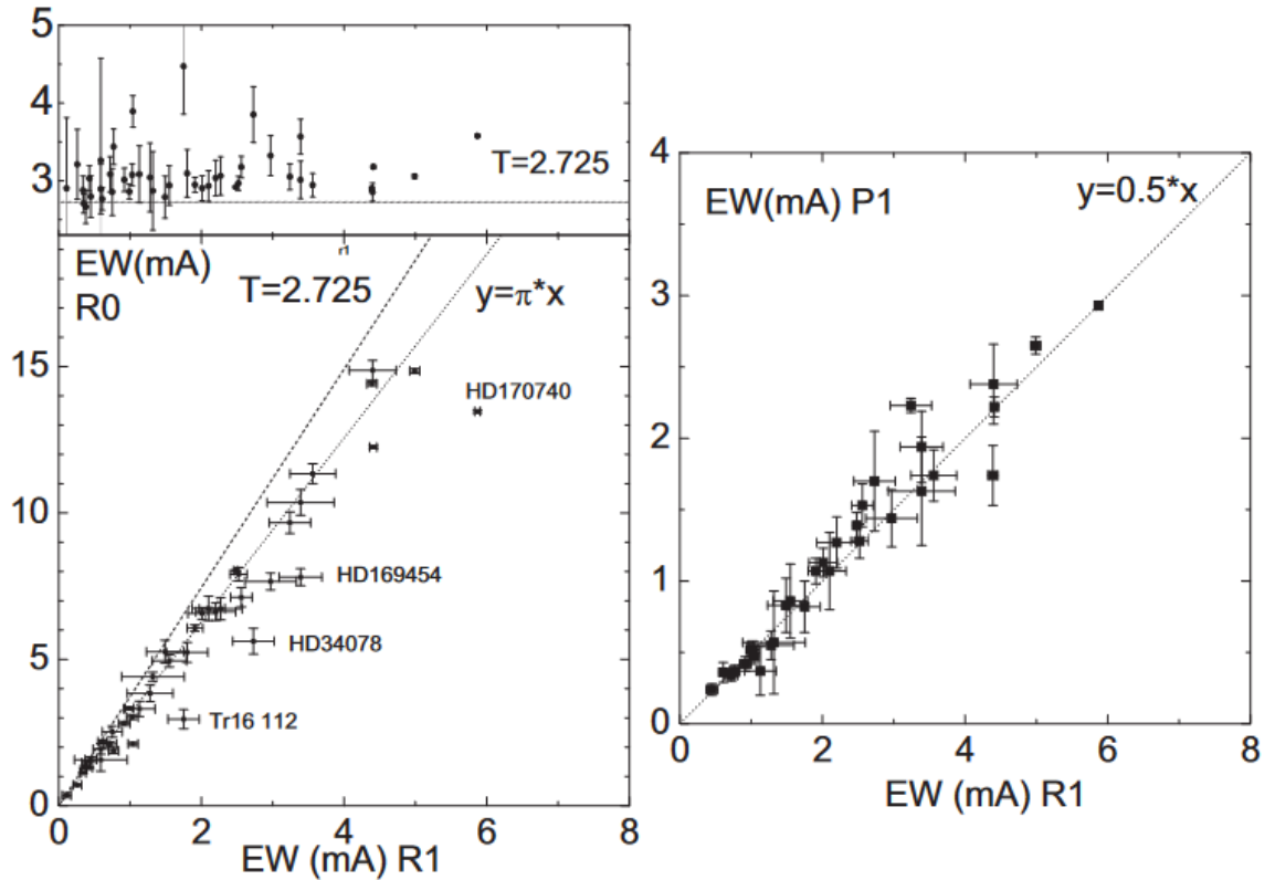
Рисунок 3.29. Эквивалентные ширины линий R(1), R(0) и P(1) полосы В-Х (0-0) CN из работы Krelowski et al. (2012). Значения T_{\text{rot}} , отображенные на верхнем графике, основаны на лучевой концентрации, рассчитанной без учета эффекта насыщения. Все они выше температуры 2.725 К, отмеченной пунктирной горизонтальной линией. Пунктирная линия на нижнем левом графике показывает отношение эквивалентных ширин R(0)/R(1) при T_{\text{rot}} = 2.725 К и отношение сил осцилляторов из Roth & Meyer (1995). Отношение эквивалентных ширин линий P(1) и R(1) (0,5) соответствует указанным выше параметрам.
