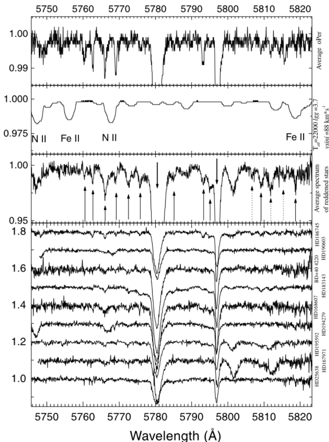
Рисунок 5.3. Фрагмент обзора Galazutdinov et al. (2000a). Показаны диффузные межзвездные полосы, наблюдаемые в спектре HD 23180 (верхняя часть рисунка) и в спектрах сильно покрасневших звезд (нижняя часть). Другие части (как подписано справа) показывают синтетический спектр для HD 23180 и средний спектр для всех покрасневших звезд в межзвездной шкале длин волн. Стрелки показывают положение ДМП. Сплошные стрелки — это ДМП, известные ранее, пунктирные стрелки — новые ДМП, обнаруженные в обзоре (Galazutdinov et al. 2000a).
