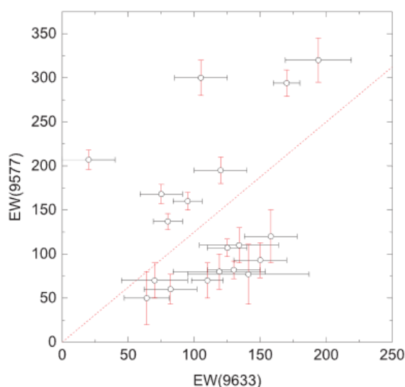
Рисунок 5.83. Сравнение эквивалентных ширин ДМП 9633 и 9577 Å. Пунктирная линия соответствует лабораторному отношению интенсивностей ДМП9633/ДМП9577 = 0.8. Разброс данных существенно выше ошибок измерений.
